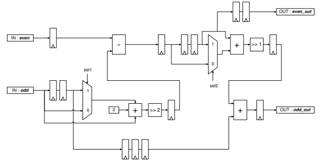
Fig. 8. Horizontal inverse DWT.
