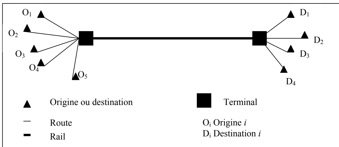
Figure 2.3. Consolidation point à point.
