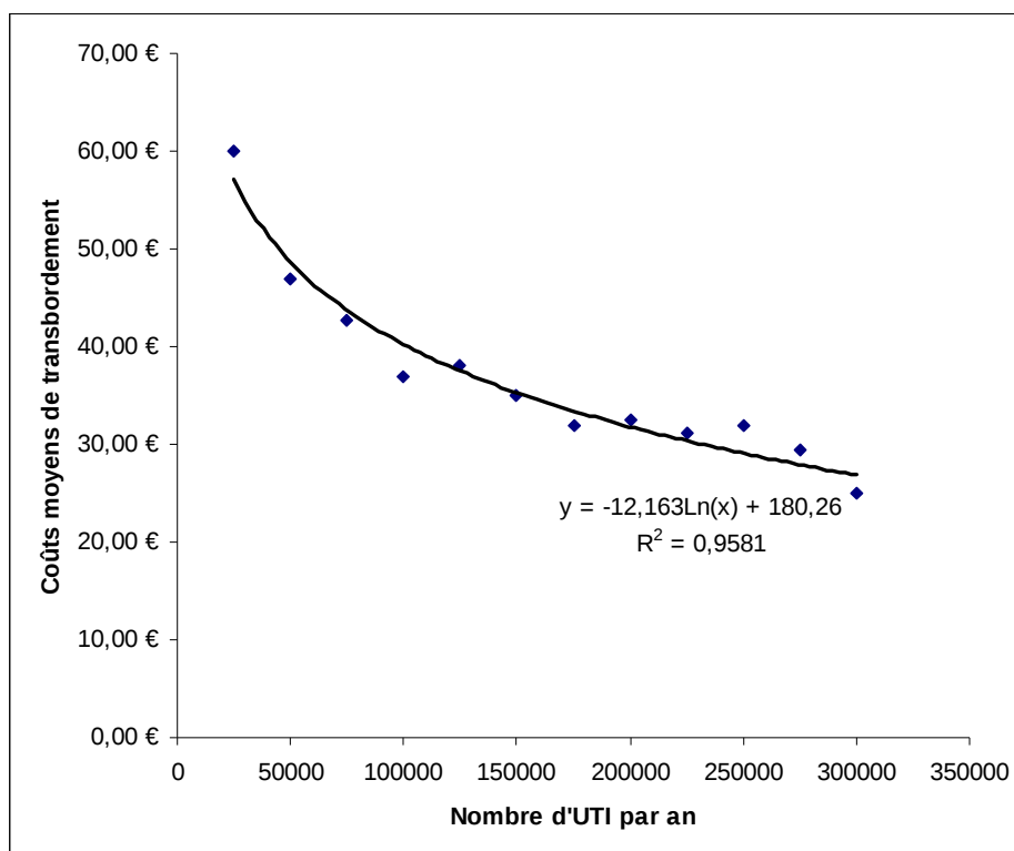
Figure 2.8. Evolution du coût moyen de transbordement en fonction du flux.
