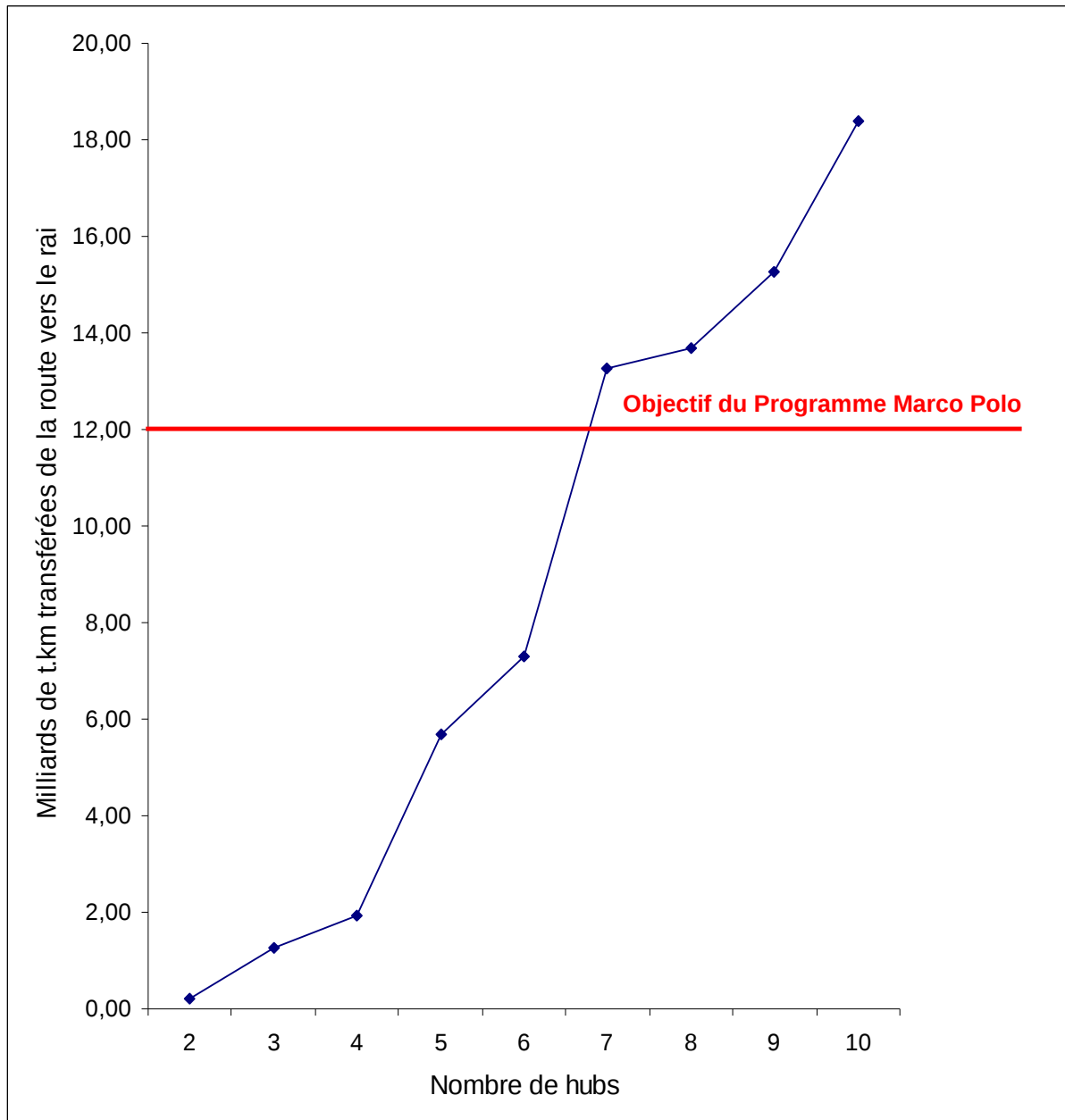
Figure 6.17. Evolution des flux transférés de la route vers le rail en fonction du nombre de hubs.
