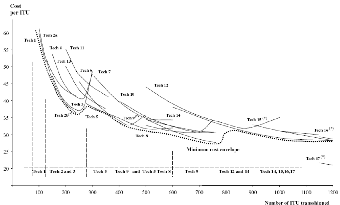
Figure 2.7. Analyse comparative du coût pour des différentes conceptions de terminaux.
