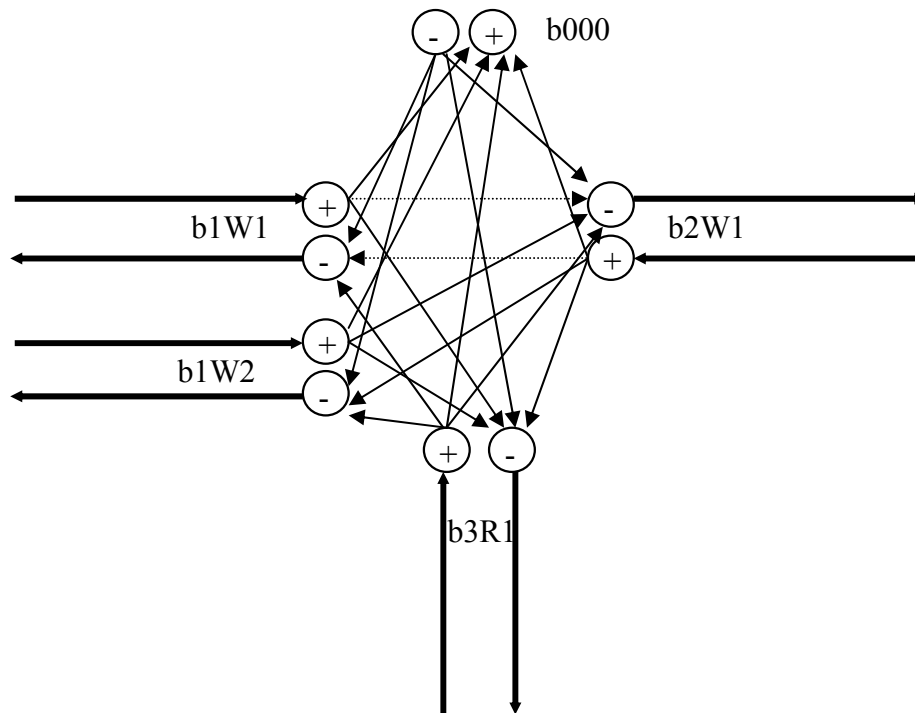
Figure 4.4. Réseau virtuel détaillé au nœud b.
