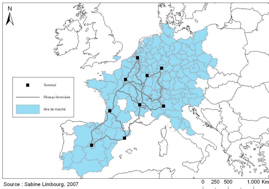
Figure A4.1. Réseau ferroviaire inter-hub et aire de marché pour une configuration à neuf hubs.
