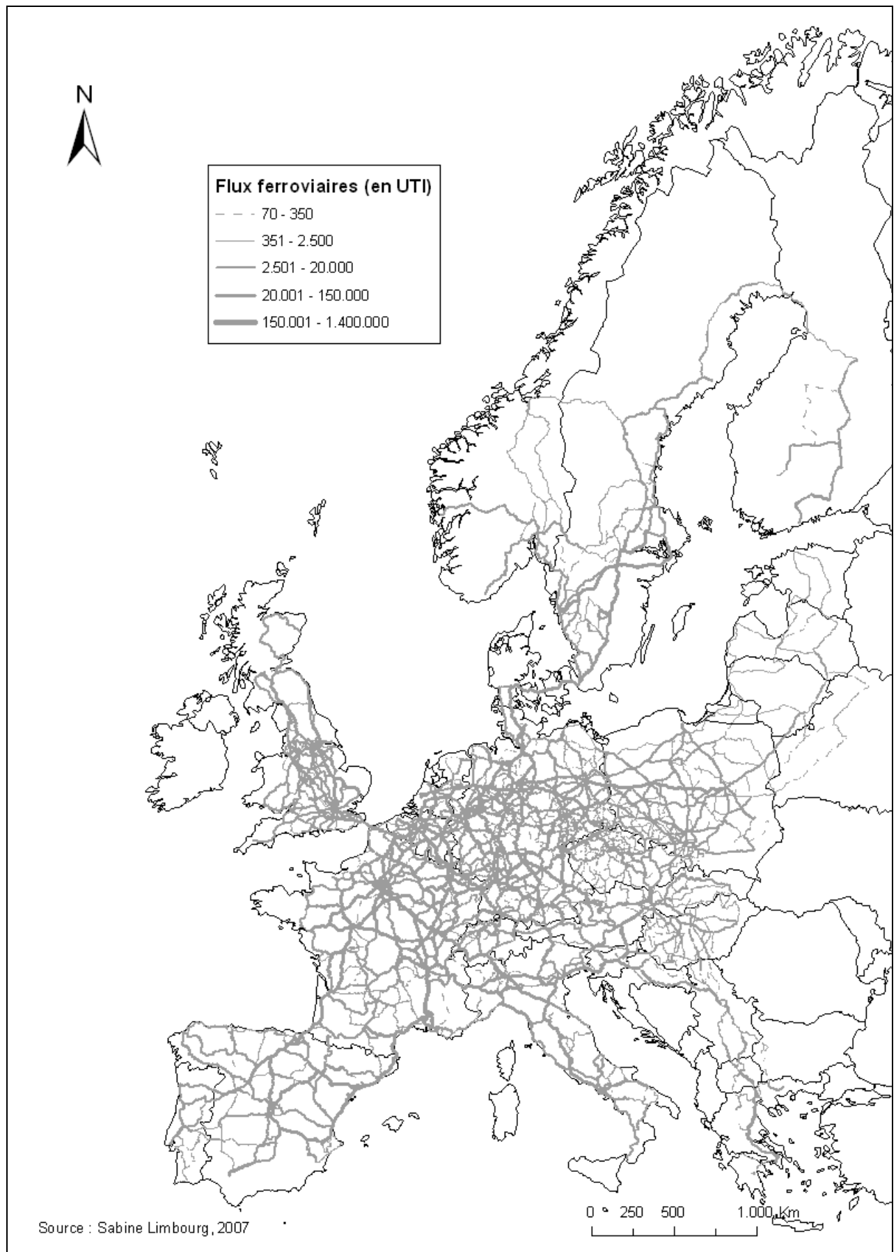
Figure 4.14. Affectation multi-flux pour le chapitre 9 et pour des déplacements de plus de 300 km sur le réseau ferroviaire.
