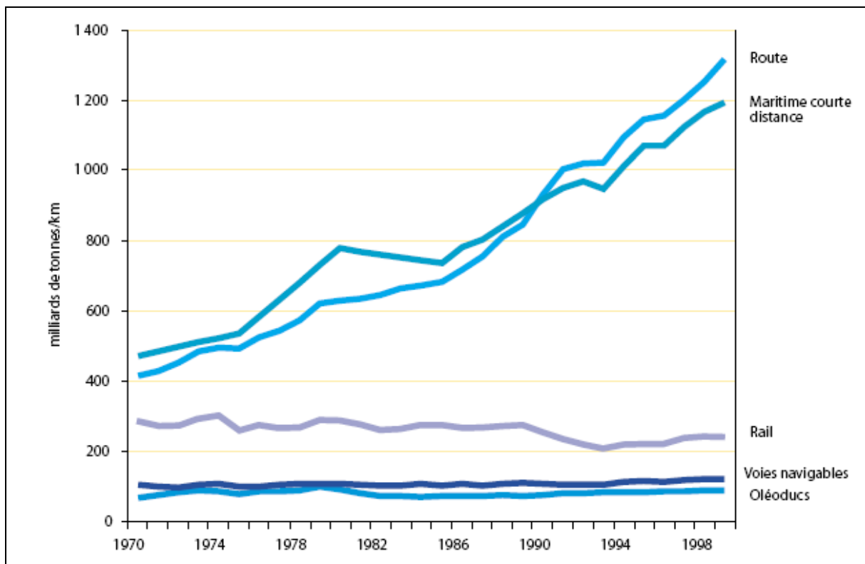
Figure 1.1. Transport de marchandises - Évolution du trafic par mode de transport EU-15 (1970-1999). Source : Livre Blanc 2001
