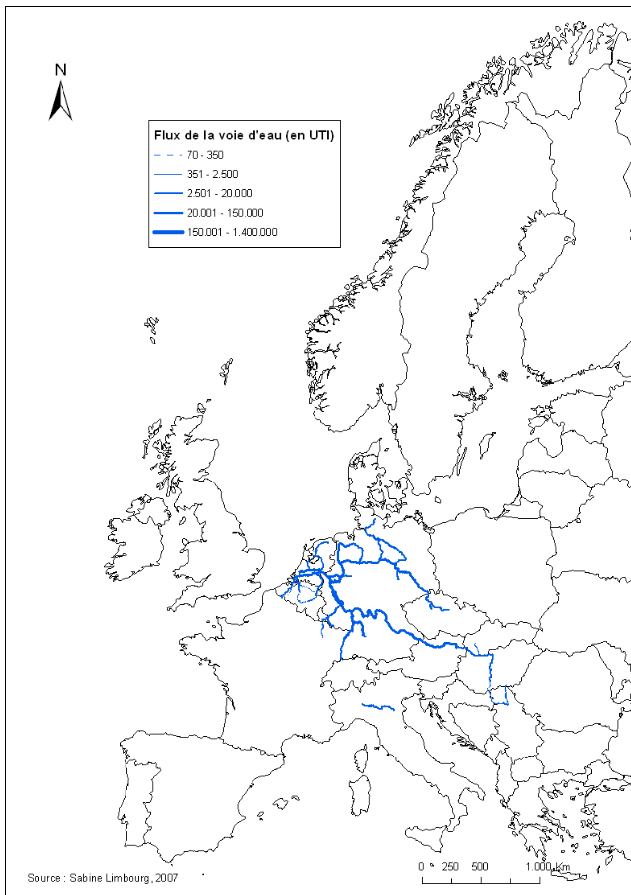
Figure 4.15. Affectation multi-flux pour le chapitre 9 et pour des déplacements de plus de 300 km sur le réseau fluvial.
