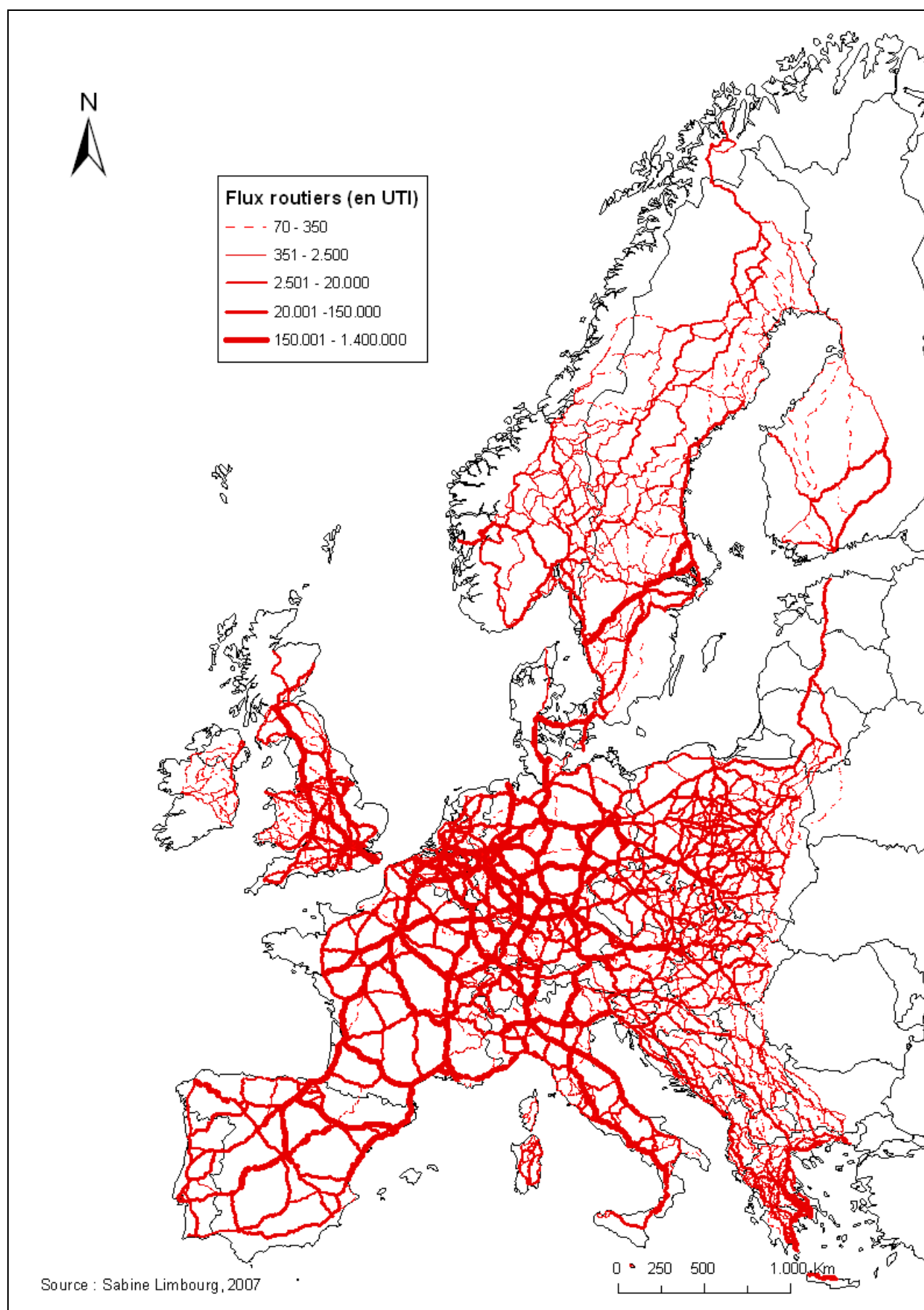
Figure 4.13. Affectation multi-flux pour le chapitre 9 et pour des déplacements de plus de 300 km sur le réseau routier.
