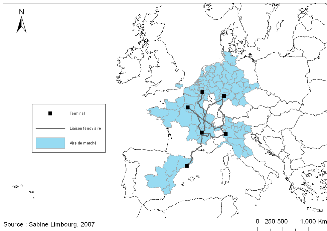
Figure 6.12. Réseau ferroviaire inter-hub et aire de marché pour une configuration à six hubs
