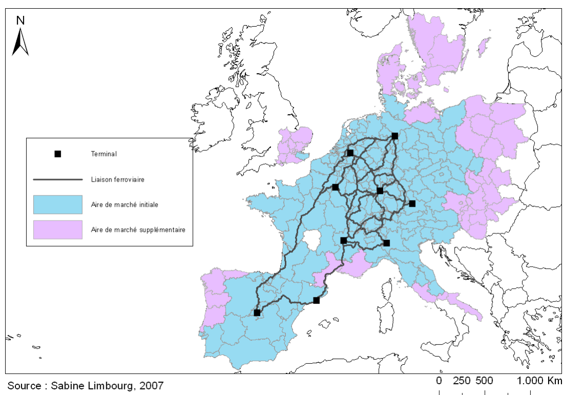
Figure A5.1. Réseau ferroviaire inter-hub et aire de marché pour une configuration à huit hubs en tenant compte des coûts externes.
