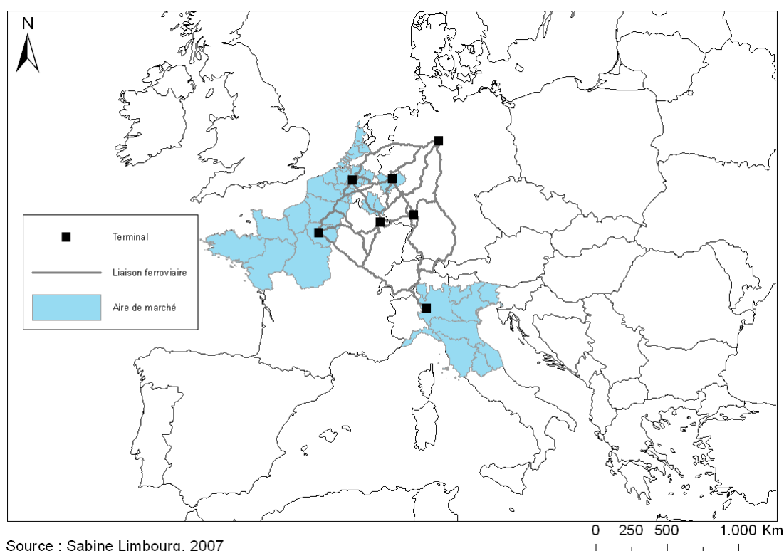
Figure 6.15. Réseau ferroviaire inter-hub et aire de marché de la configuration à sept hubs proposée par Ballis.
