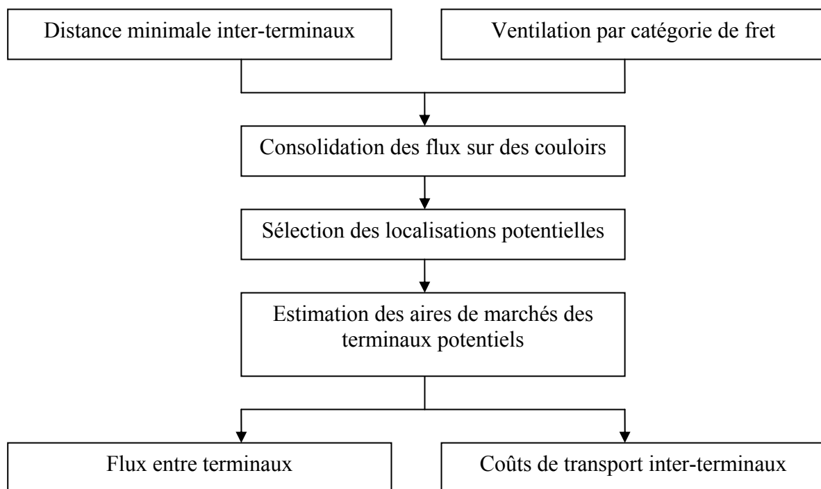
Figure 5.10. Détermination des localisations potentielles.
