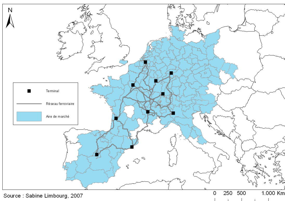
Figure A4.2. Réseau ferroviaire inter-hub et aire de marché pour une configuration à dix hubs.
