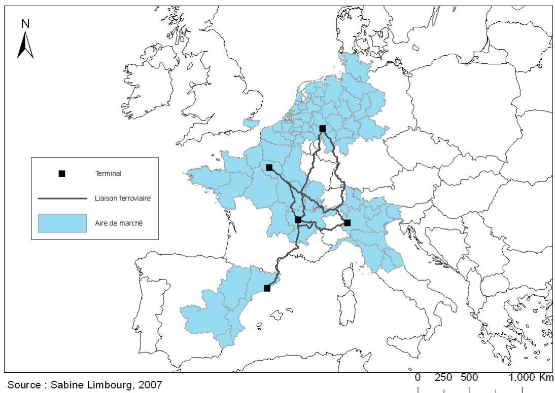
Figure 6.8. Aire de marché lorsque cinq hubs sont localisés.
