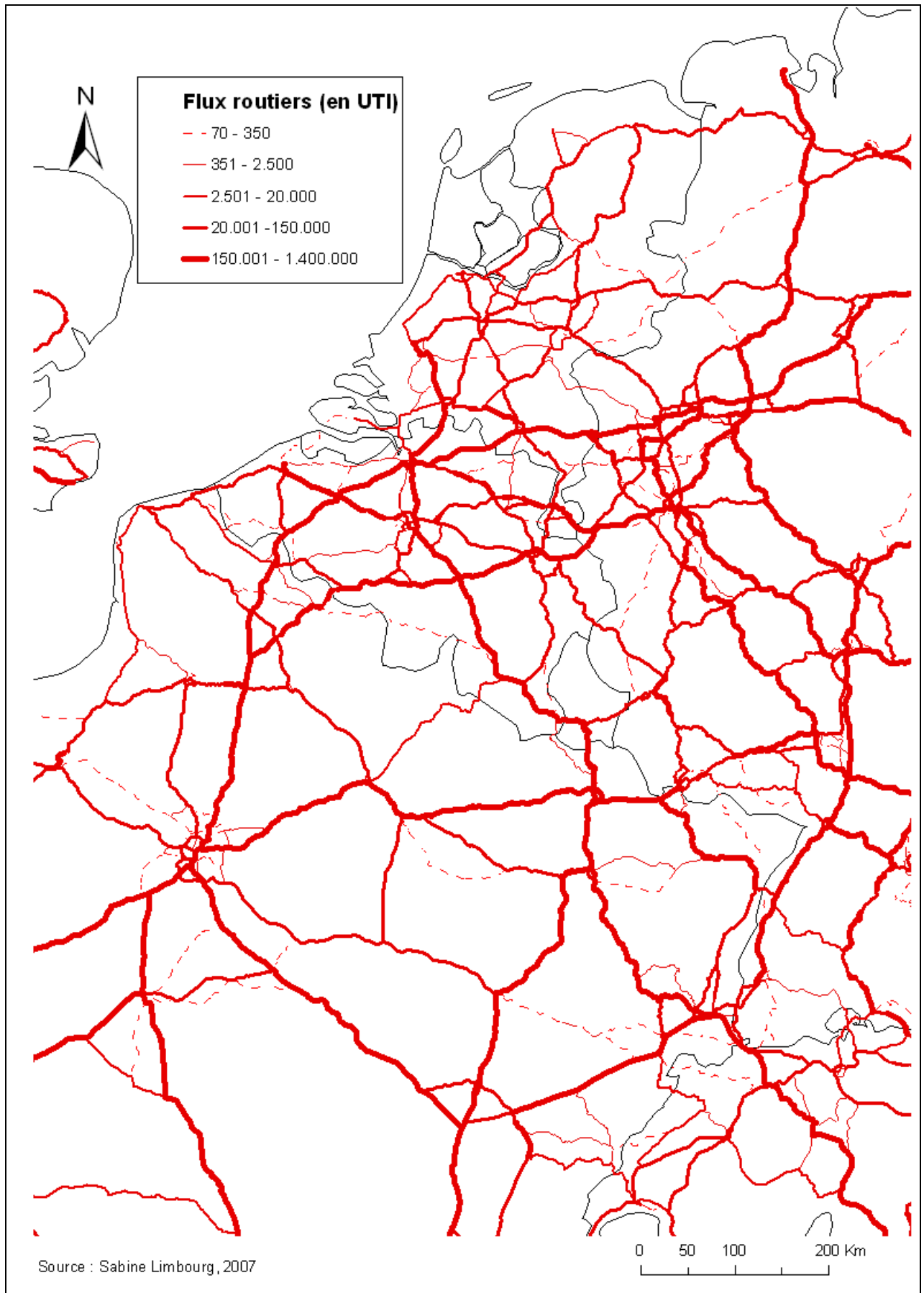
Figure 4.12. Affectation multi-flux pour le chapitre 9 et pour des déplacements de plus de 300 km sur le réseau routier du Benelux.
