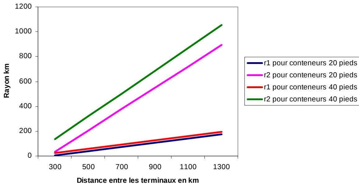
Figure 5.22. Evolution des rayons des aires de marché en fonction de la distance entre les terminaux.
