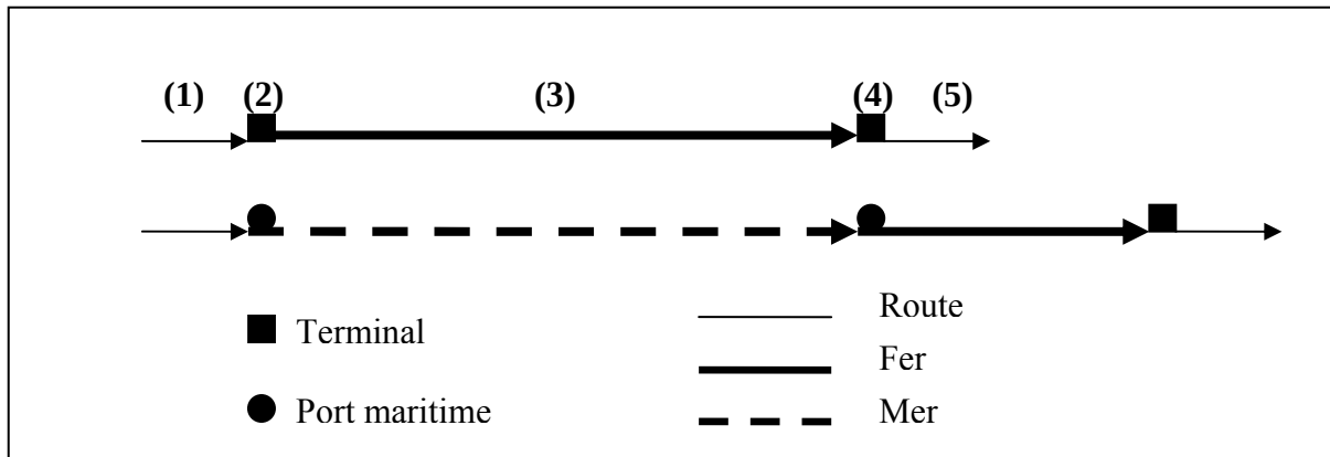
Figure 2.1. Exemples de chaîne de transport.
