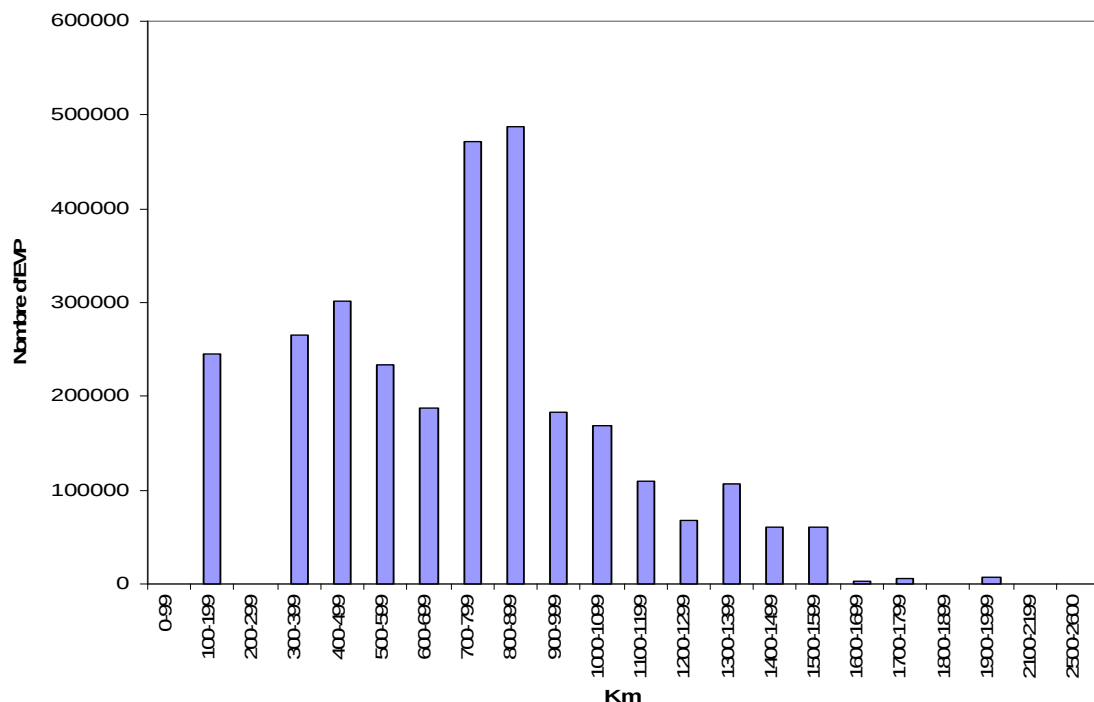
Figure 5.11. Distribution des EVP en fonction de l'éloignement des terminaux.
