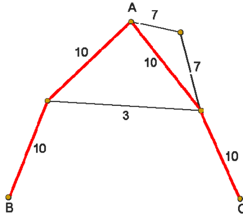
Figure 4.6. Un arbre de Dijkstra calculé à partir de A.
