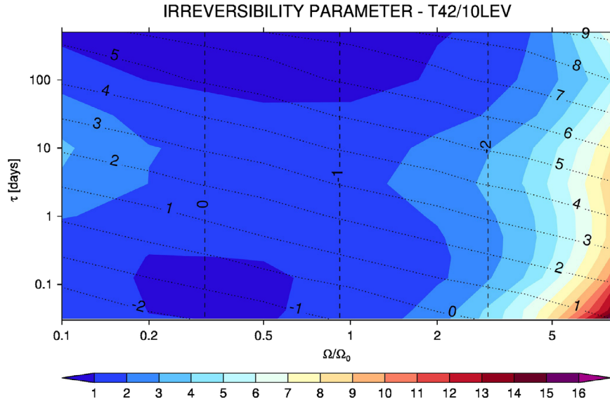
Fig. 11. Irreversibility parameter \alpha .
