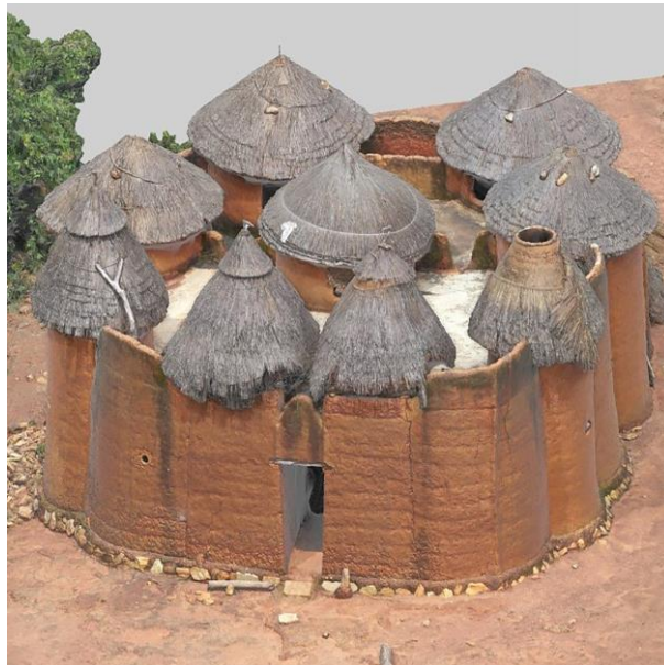
Figure 2 : Takienta typique, 2019 (photogrammétrie : Yves Baudot, Fabrice Noukpakou).
