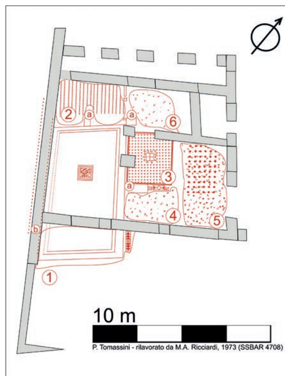
Fig. 3. Plan des structures julio-claudiennes retrouvées en 1973.
