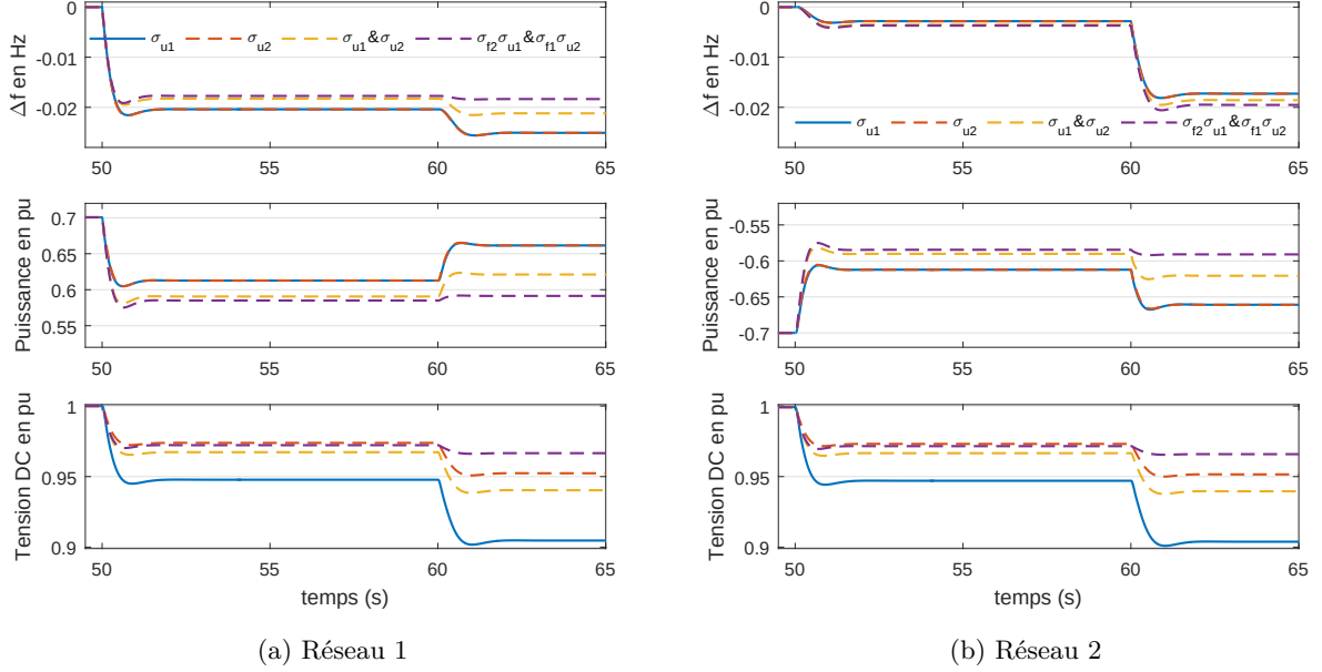
Figure 4.8 – Scénario 4 : perte de production de 300MW dans la zone 1 à t=50s et de 500MW dans la zone 2 à t=60s, comparaison entre la réponse du système pour différentes valeurs du statisme de tension et de fréquence
