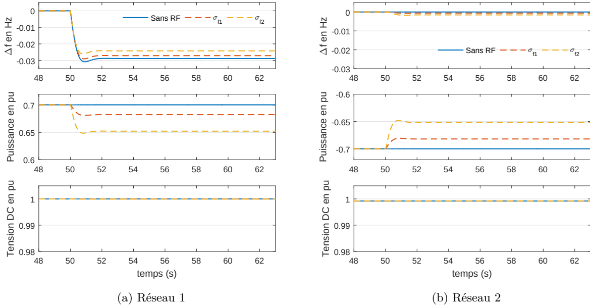
Figure 4.6 – Scénario 3 : perte de production de 300MW dans la zone 1 à t=50s , réponse du système sans réglage de fréquence et avec réglage (pour deux valeurs de statistisme)
