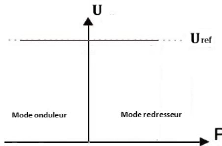
Figure 3.4 – Caractéristique U - P du contrôleur de la tension DC
