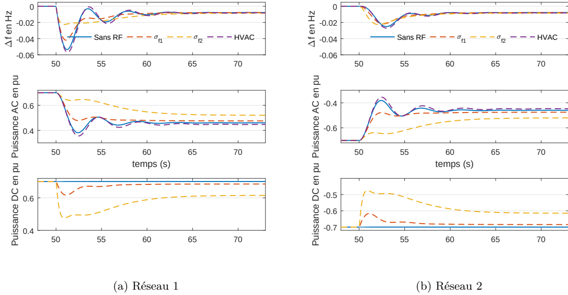
Figure 4.13 – Réponse d'un système à deux zones reliées par une ligne AC parallèle à un lien HVDC suite à la perte de 300 MW de production dans la zone 1 : comparaison entre HVAC sans réglage de fréquence et avec réglage.
