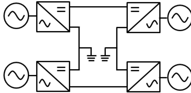
Figure 2.7 – Liaison bipolaire
