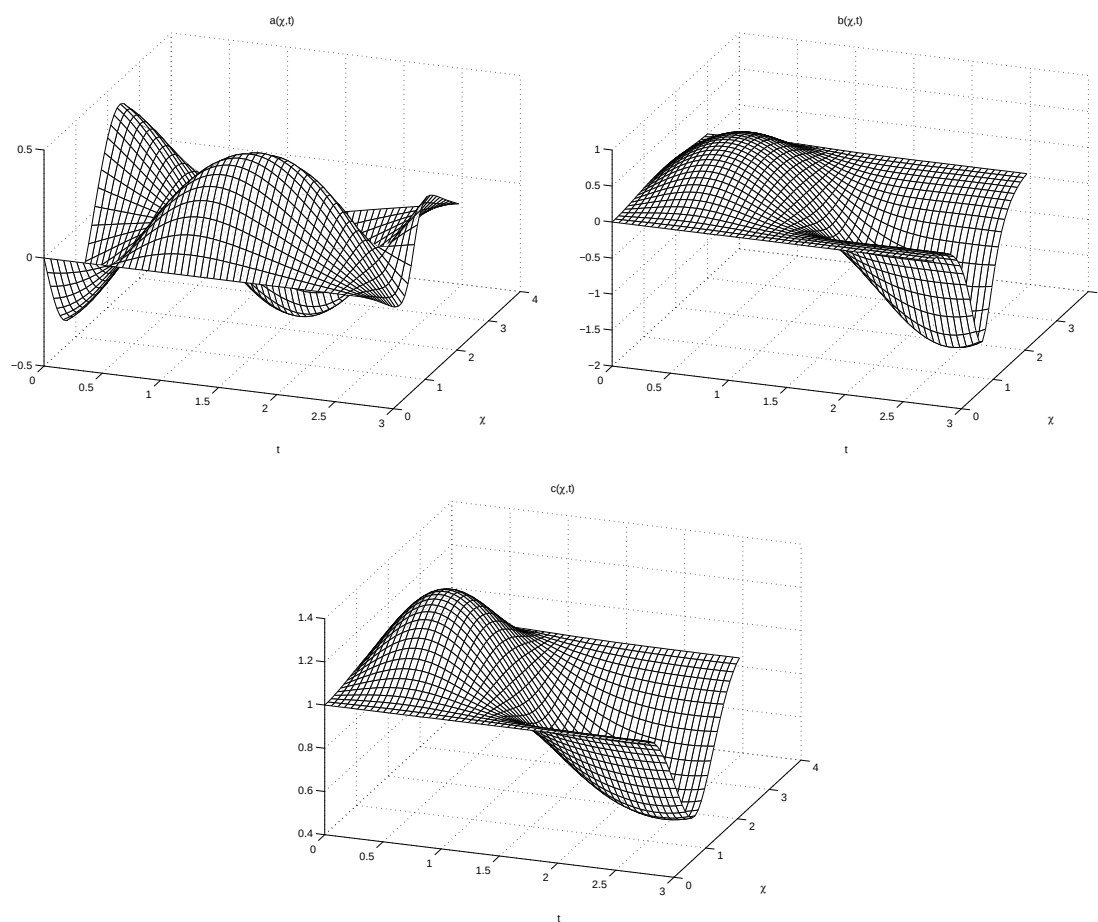
Figure 2.8 – Composantes temporelle, radiale et angulaire a , b , c des champs de jauge pour la particule oscillant dans autour du minimum topologique de la Figure 2.7 (univers fermé)
