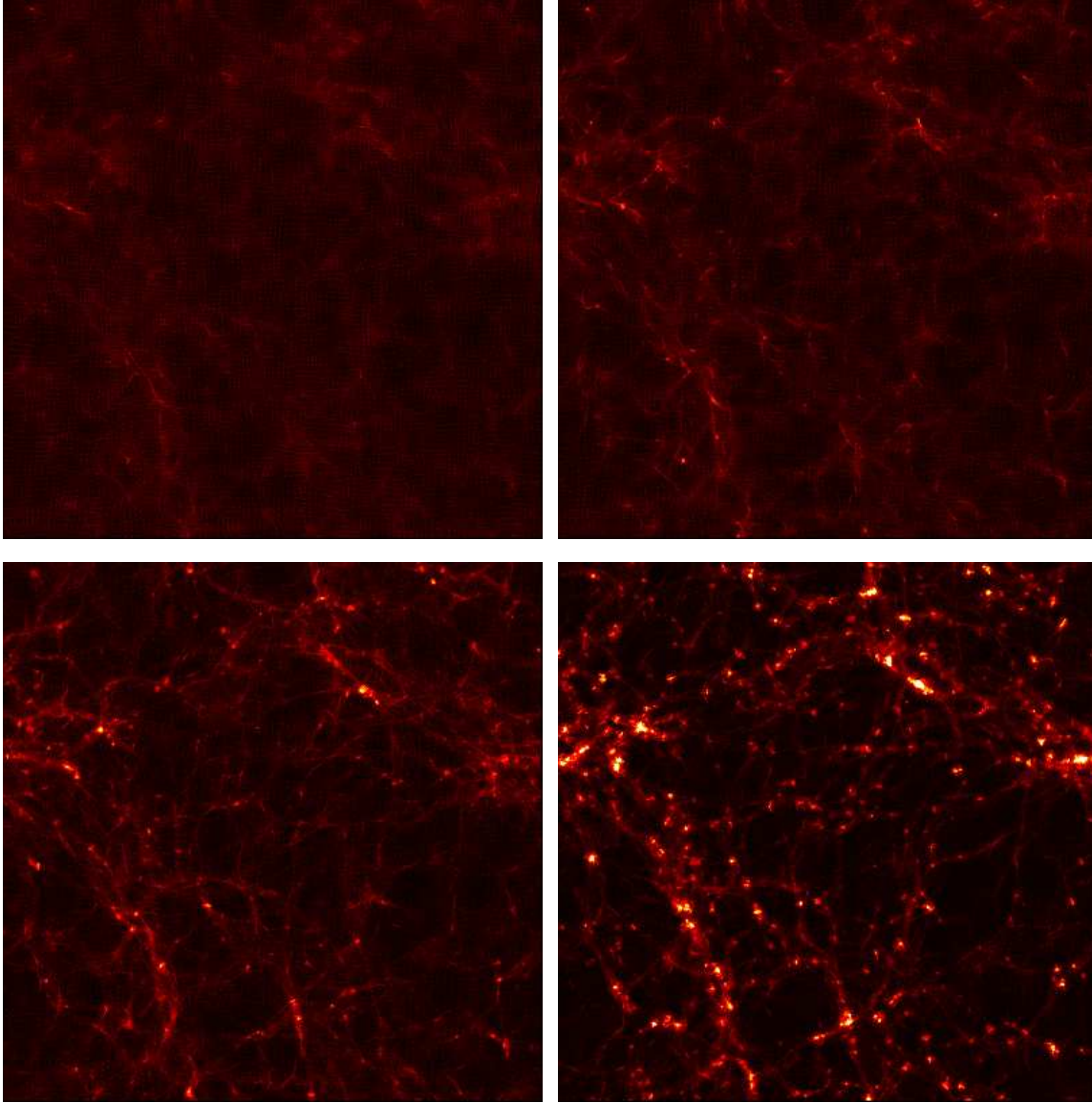
Figure 7.12 – Champs de densité des 128^3 particules dans un cube de longueur d'arête valant 128h^{-1}\text{Mpc} , projetées dans le plan (x, y) , à différents redshifts z pour le modèle à constante cosmologique (de gauche à droite et de haut en bas : z = 3 , z = 2 , z = 1 , z = 0 )
