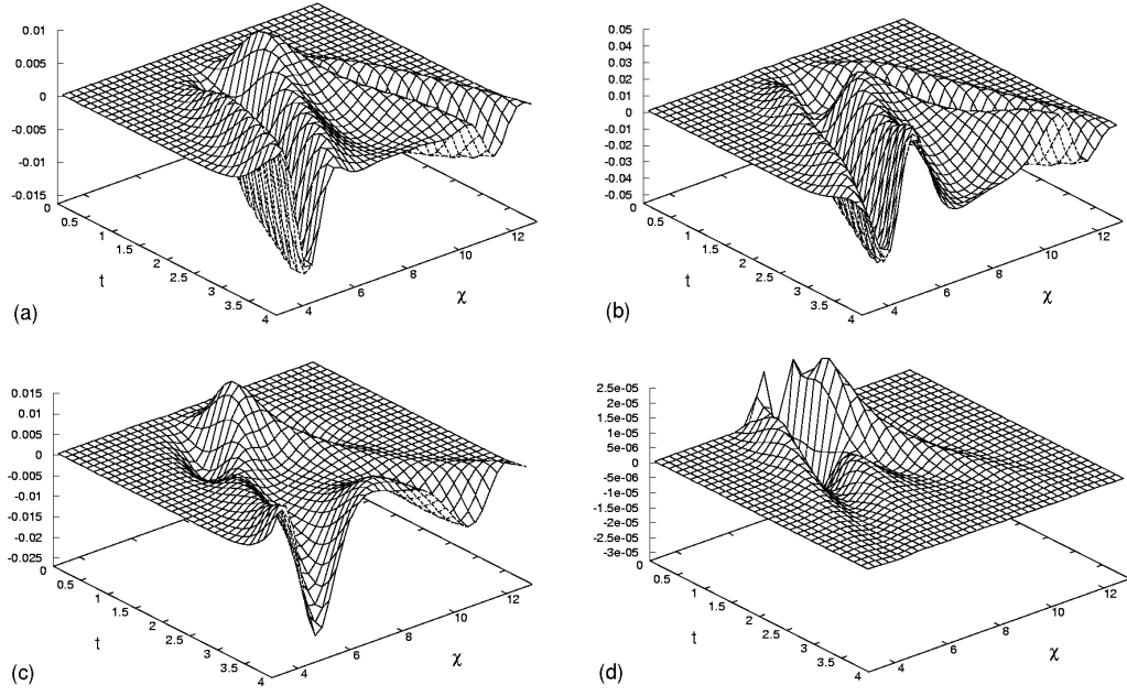
Figure 4.4 – Contrastes de densité et de pressions, ainsi que la composante non diagonale du tenseur énergie-impulsion : (a) \frac{-T_0^0}{\rho_B^0} - 1 (b) \frac{3T_1^1}{\rho_B^1} - 1 (c) \frac{3T_2^2}{\rho_B^2} - 1 (d) -T_0^1 (mêmes paramètres qu'à la figure 4.1)
