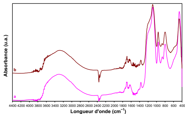
Fig. 10. Spectres DRIFT du \text{PMo}_{11}\text{V}/\text{HMS} avant (a) et après (b) test catalytique pendant cinq heures à 350\text{ }^{\circ}\text{C} .
