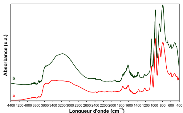
Fig. 9. Spectres DRIFT du \text{PMo}_{11}\text{V} avant (a) et après (b) test catalytique pendant cinq heures à 350\text{ }^{\circ}\text{C} .
