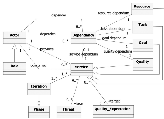
GI-Tropos Meta-model
