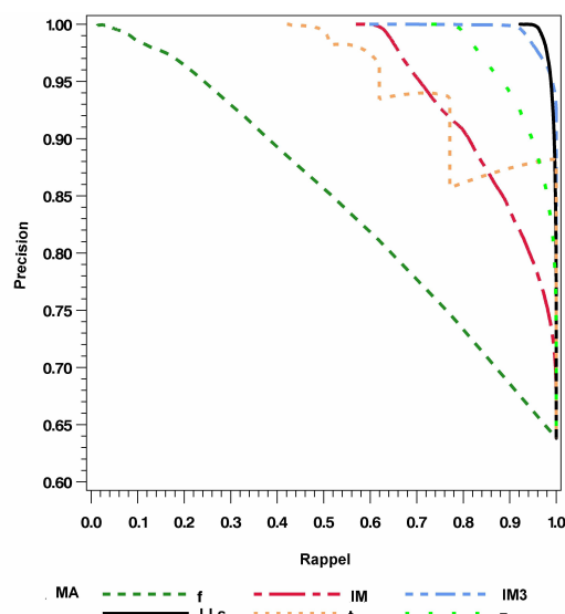
FIGURE 2 – Courbes PR pour les trigrammes
