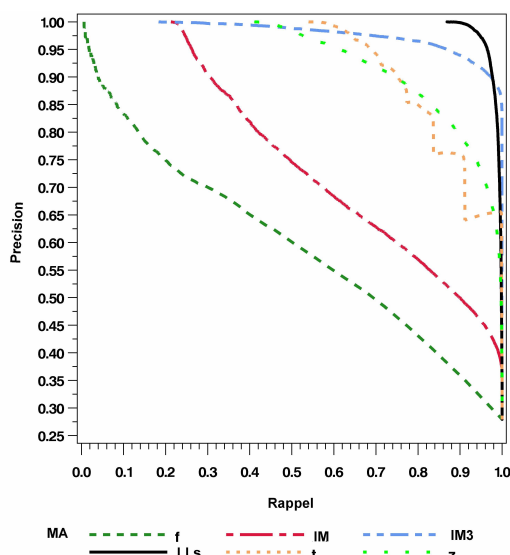
FIGURE 1 – Courbes PR pour les bigrammes
