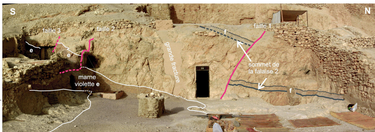
FIG. 11. Exemple de failles sur la façade de la TT 29.
