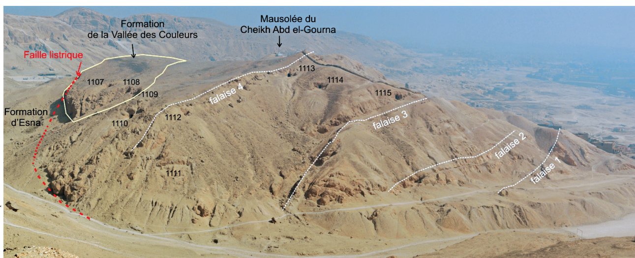
FIG. 10. Disposition des unités lithologiques sur le versant sud-ouest de la colline de Cheikh Abd el-Gourna, vers la Vallée des Couleurs. Position de quelques tombes MMA.
