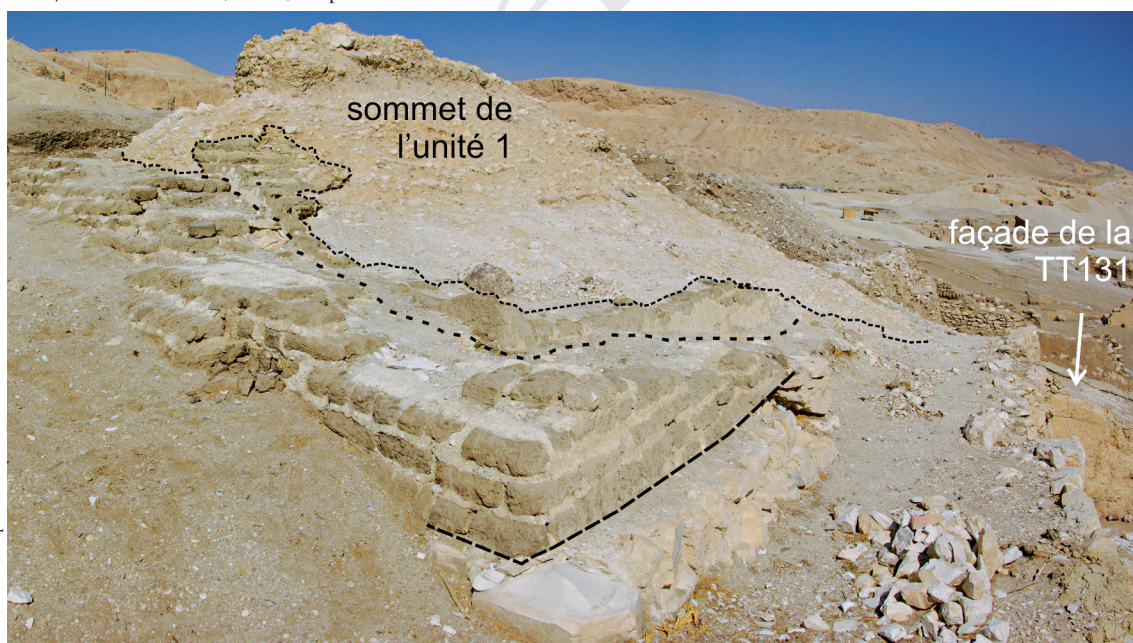
FIG. 8. Pyramide aménagée sur le rebord de la falaise 1 et incorporant un chicot rocheux du sommet de l'unité 1 du Calcaire de Thèbes, au-dessus de la TT 131. Les tirets longs indiquent la base de la construction et les tirets les plus fins, l'interface entre les briques crues et la roche en place. Entre les deux on discerne les traces d'enduit qui délimitent une première étape de la construction de la superstructure.
