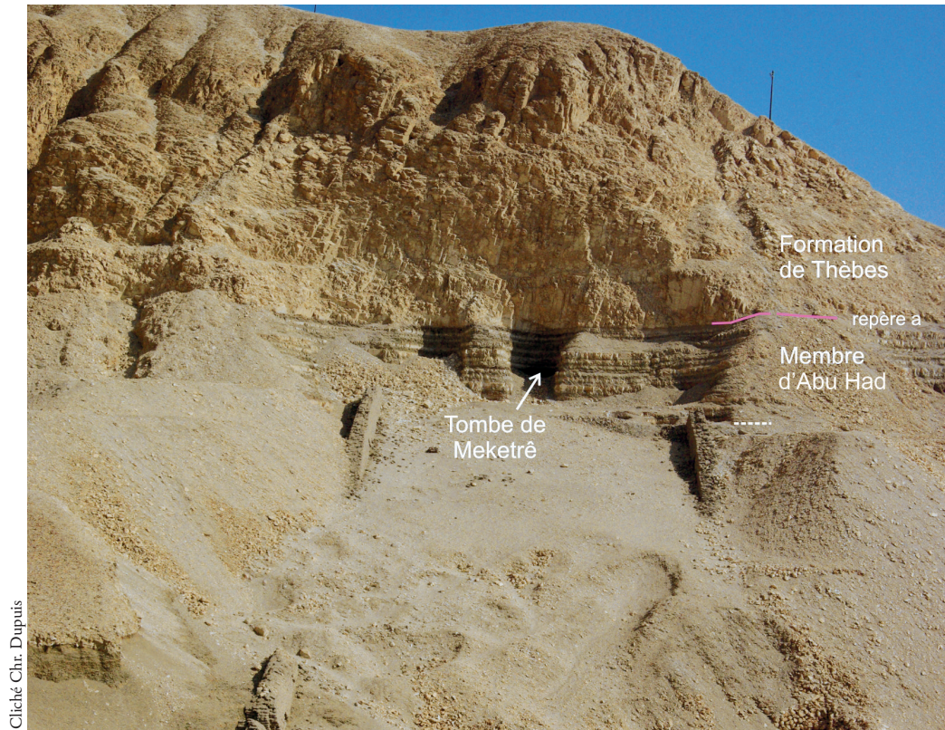
FIG. 17. Entrée de la tombe de Meketrê (TT 280/MMA 1101) creusée dans le sommet des Marnes d'Esna (Membre d'Abu Had), quelques mètres sous la Formation de Thèbes.
