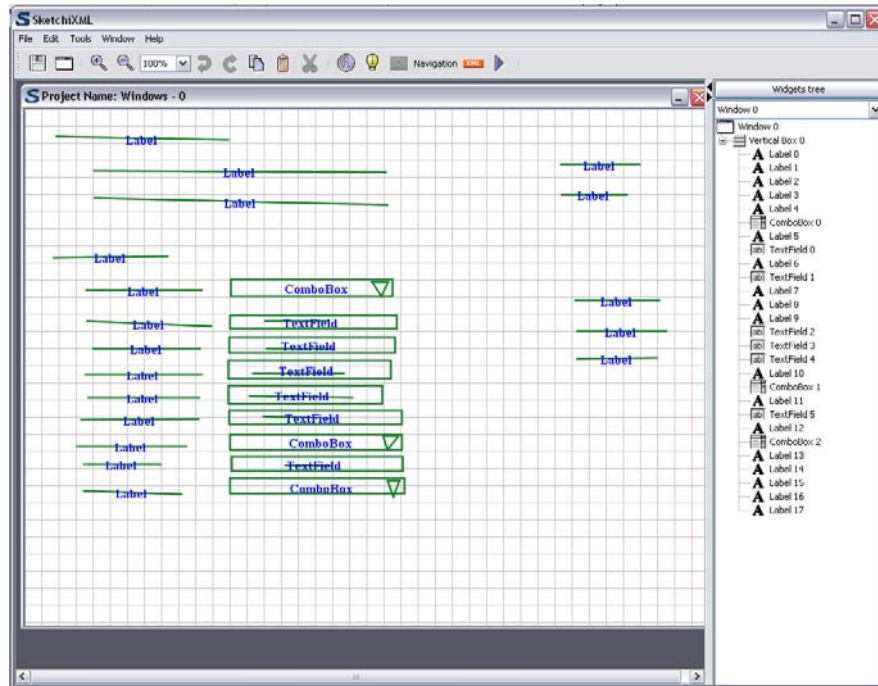
Figure 15. Interface de SketchiXML en mode de spécification de la présentation (prototypage présentationnel)
