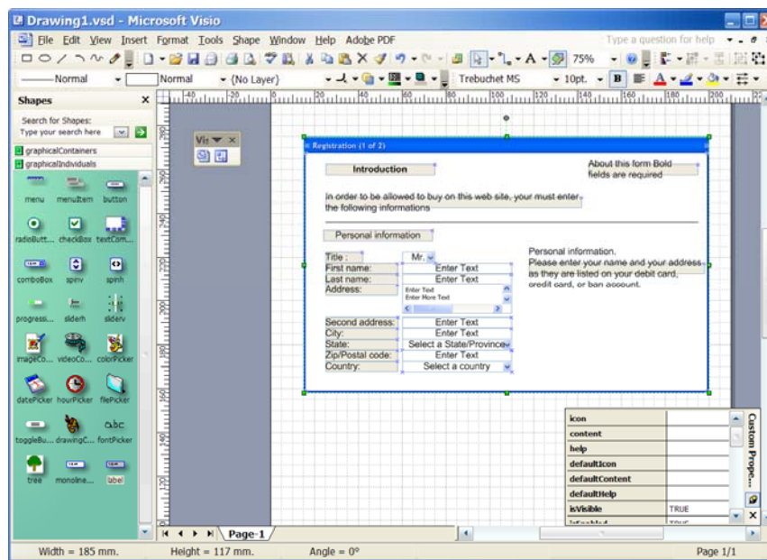
Figure 12. Interface de VisiXML en mode de spécification de la présentation (prototypage présentationnel)
