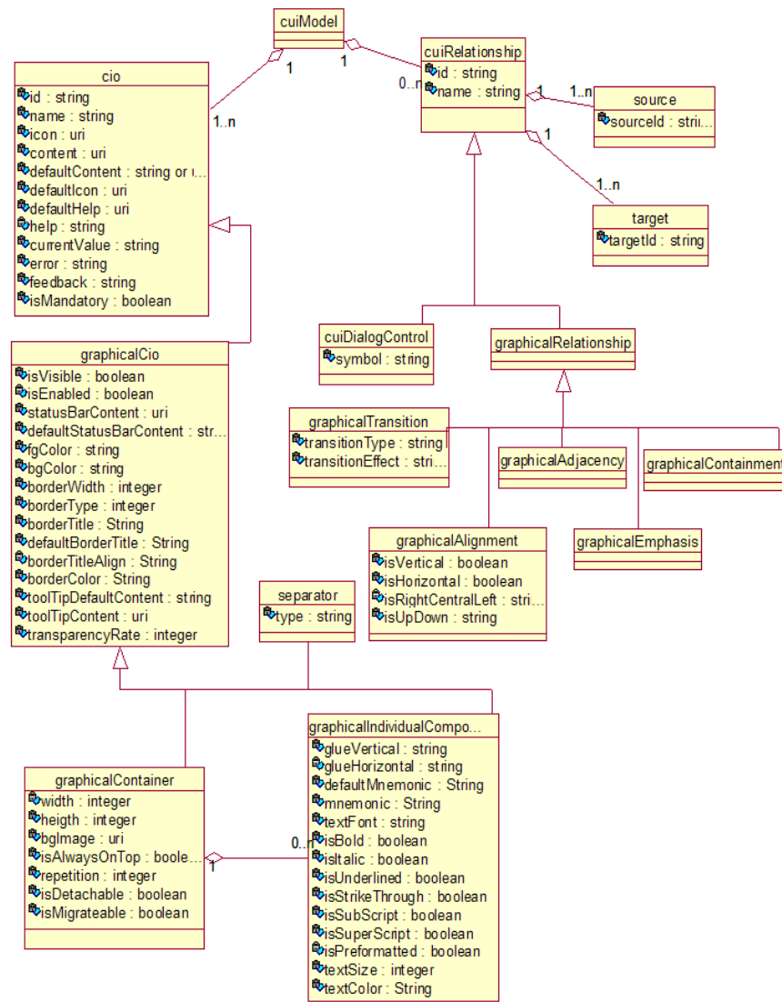
Figure 1. Méta-modèle d'une interface concrète (Limbourg et Vanderdonckt, 2004a, 2004b)
