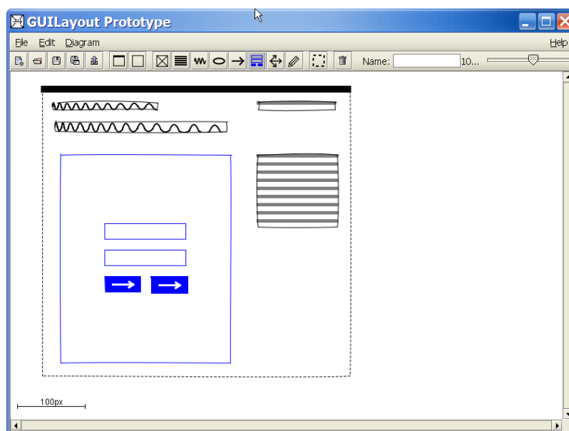
Figure 13. Interface de GUILayout en mode de spécification de la présentation (prototypage présentationnel)
