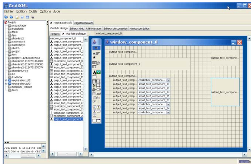
Figure 8. Interface de GrafiXML en mode de composition de la présentation (prototypage présentationnel)
