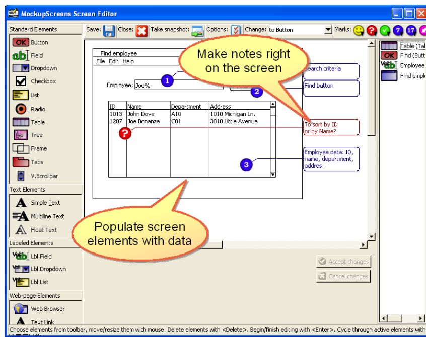
Figure 11. Interface de MockupScreens en mode de spécification de la présentation (prototypage présentationnel)
