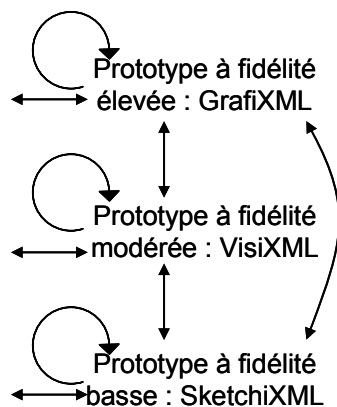
Figure 17. Trajectoires possibles de prototypages en UsiXML
