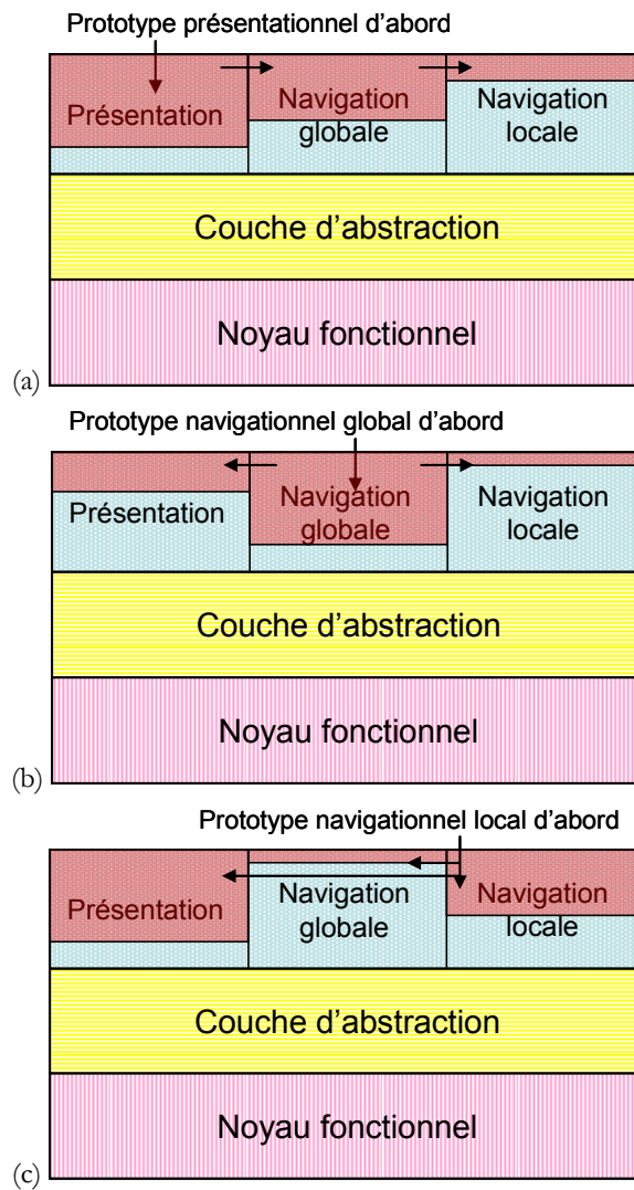
Figure 7. Différents prototypages de l'interface : « présentationnel » (a), « navigationnel global » (b), « navigationnel local » (c).
