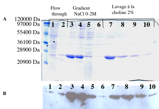
Figure 27 Analyse en SDS-PAGE et Western Blot des fractions protéiques s'éluant de la colonne DEAE-Sépharose Fast flow après application de différents tampons. Pour chaque fraction de 5 ml récoltée, 10 µl ont été déposés par piste.
