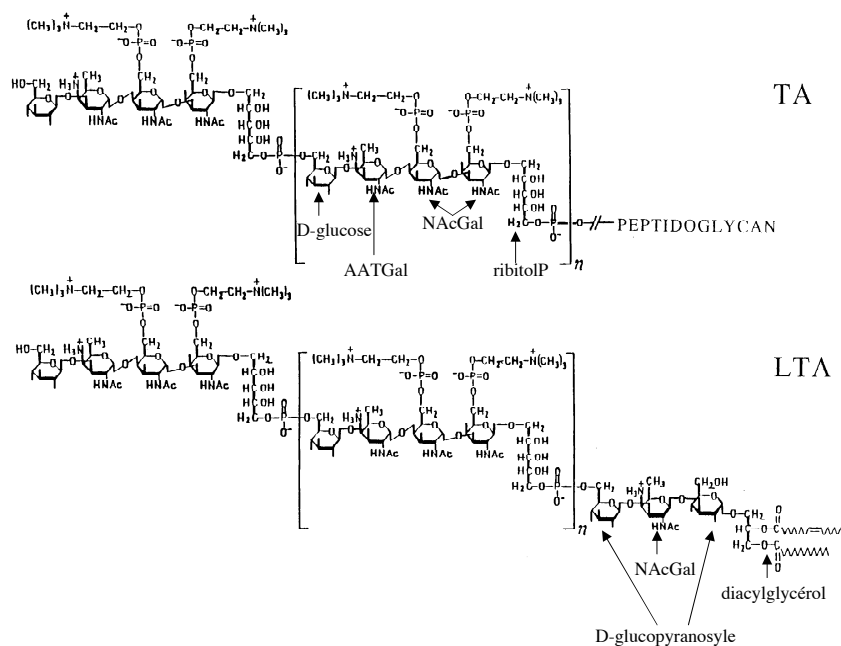
Figure 12 Structure de l'acide téichoïque (TA) et de l'acide lipotéichoïque (LTA) de la souche R6 de Streptococcus pneumoniae (modifié de (Tomasz and Werner, 2000)). TA : acide téichoïque, LTA : acide lipotéichoïque, AATGal : 2-acétamido-4-amino-2,4,6-tridéoxy-D-galactose, NacGal : N-acétyl-galactosamine.
