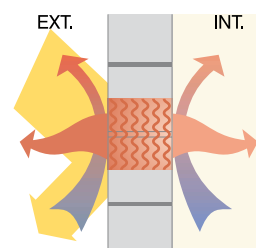
Principe de l'inertie : capacité thermique, diffusivité, effusivité.
