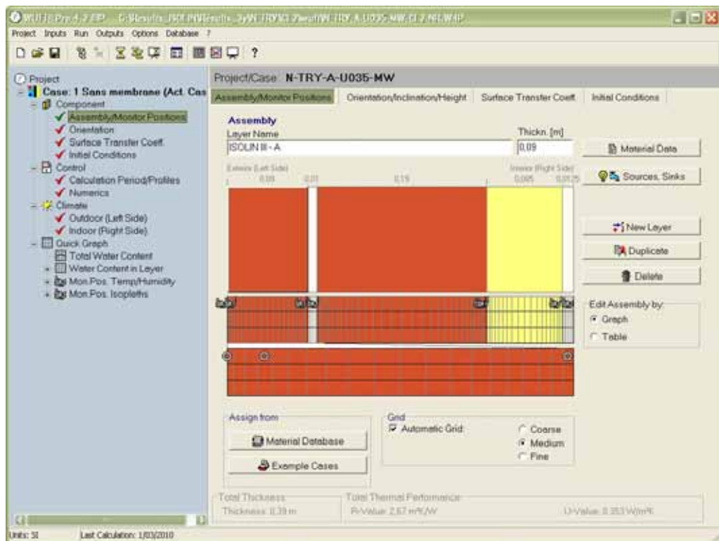
Logiciel WUFI®Pro – Encodage des données de la simulation.
