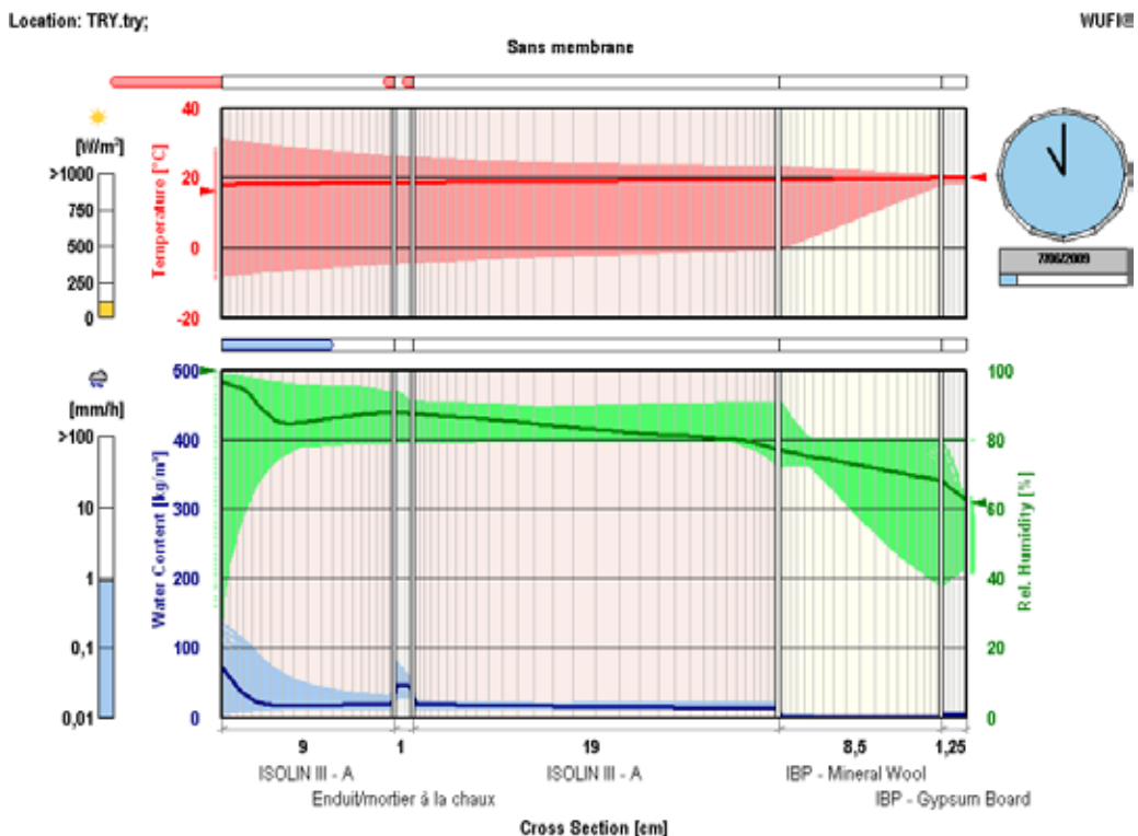
Logiciel WUFI®Pro – Visualisation des résultats sous forme de film. La courbe rouge montre la répartition de la température dans le composant à un instant donné. Les courbes verte et bleue sont corrélées, elles expriment respectivement la répartition de l'humidité relative et de la teneur en eau à travers le composant. L'interface fait aussi apparaître les flux de chaleur et d'humidité aux interfaces, ainsi que le rayonnement solaire et la quantité de pluie battante.
