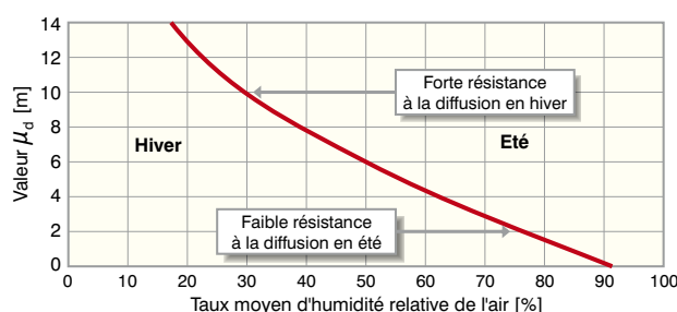
Principe de fonctionnement d'une membrane intelligente. Source : Proclima.
