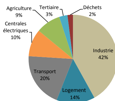
Gaz à effet de serre par secteur en Wallonie en 2004. Source : DGRNE Etat de l'environnement wallon, 2006.
