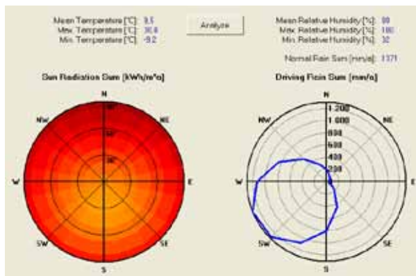
Analyse du climat à Uccle (TRY).
