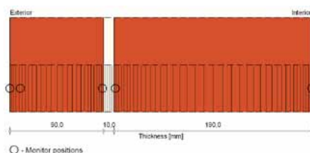
Modélisation du mur existant sur WUFI®.
