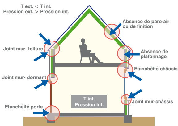
A gauche : Infiltrations d'air fréquentes dans les bâtiments. A droite : Test blower door - côté extérieur et intérieur.
