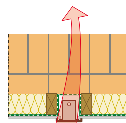
Vue en plan de l'encastrement d'une prise électrique.
