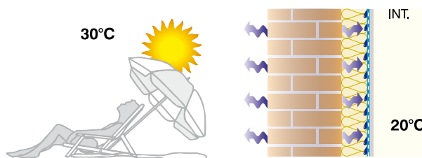
Risque de condensation interne en été si une membrane pour réguler la vapeur empêche la migration de vapeur vers l'intérieur.
