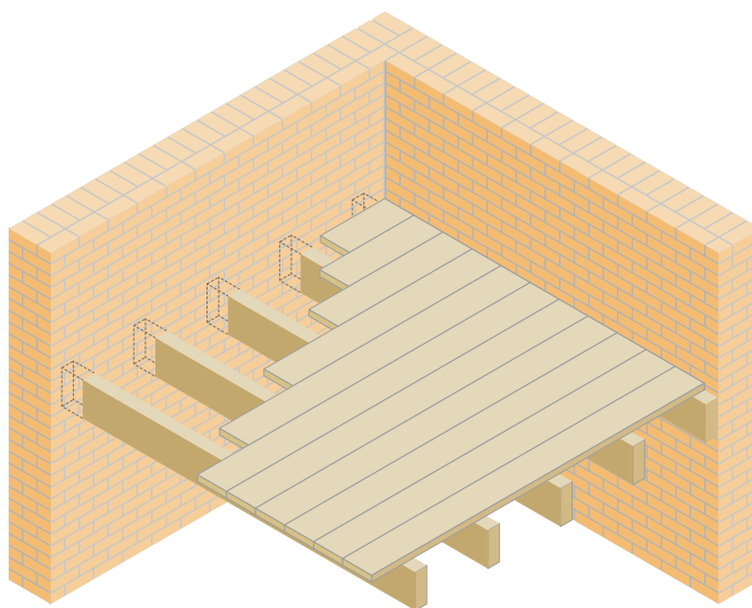
Vue d'ensemble des encastresments d'un plancher en bois dans un mur en brique avant la réalisation d'un système d'isolation par l'intérieur.
