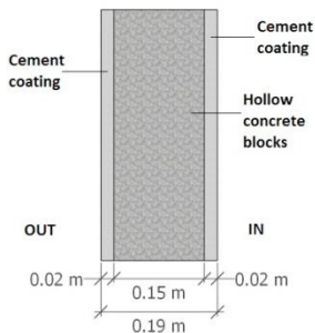
Fig. 4.a Component A: concrete wall
