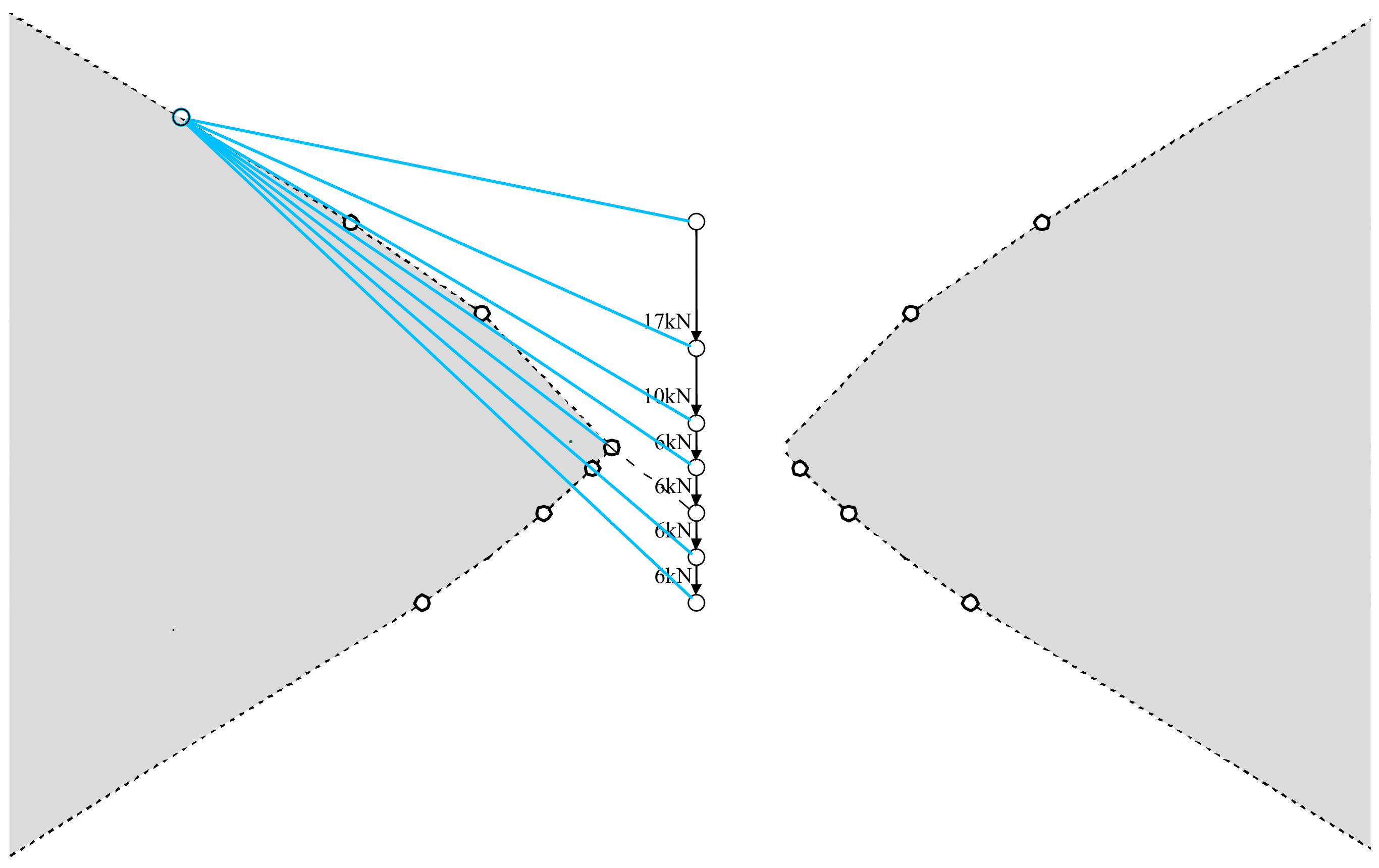
Diagramme des forces [k]
