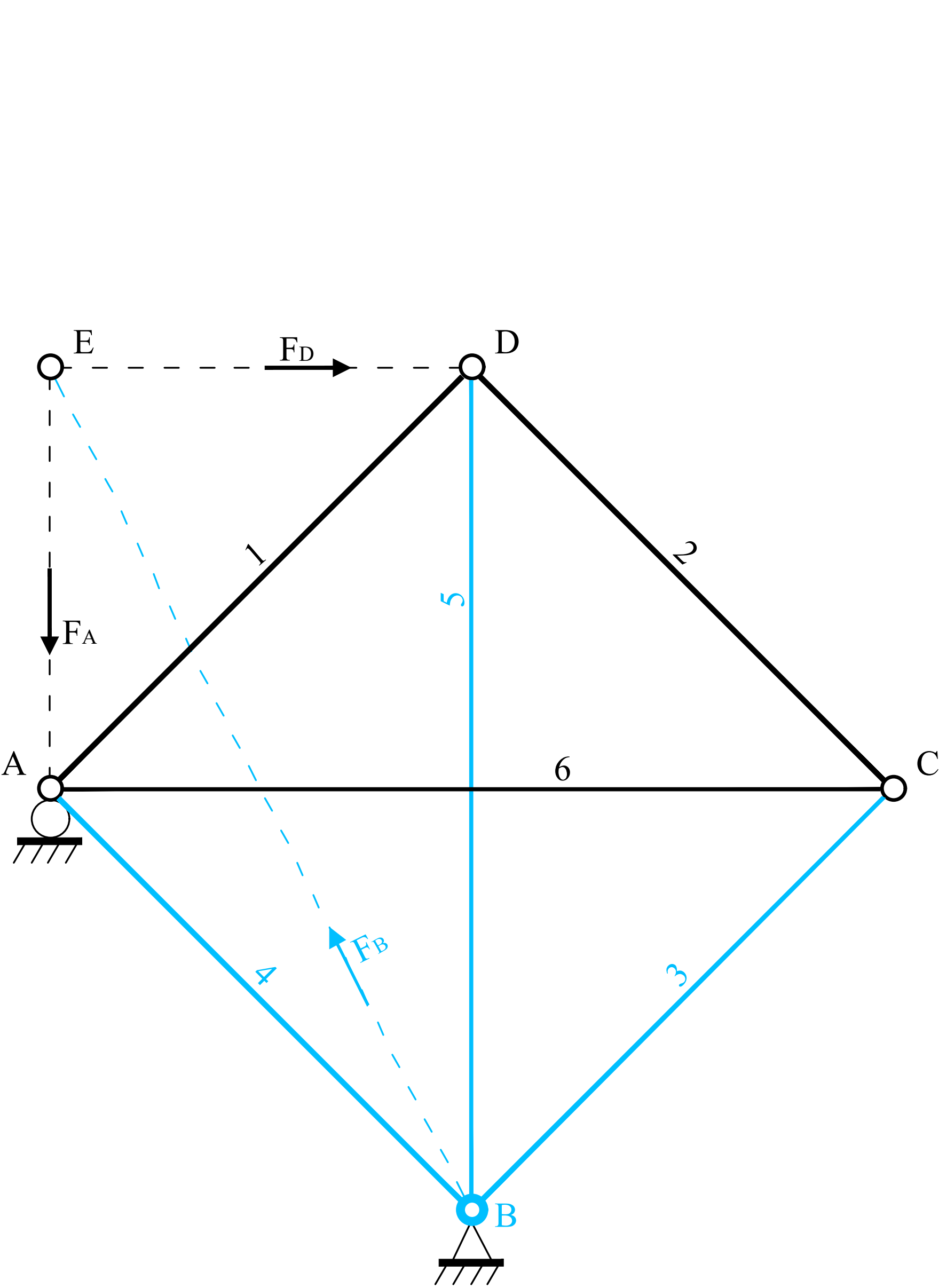
DIAGRAMME DES SITUATIONS
