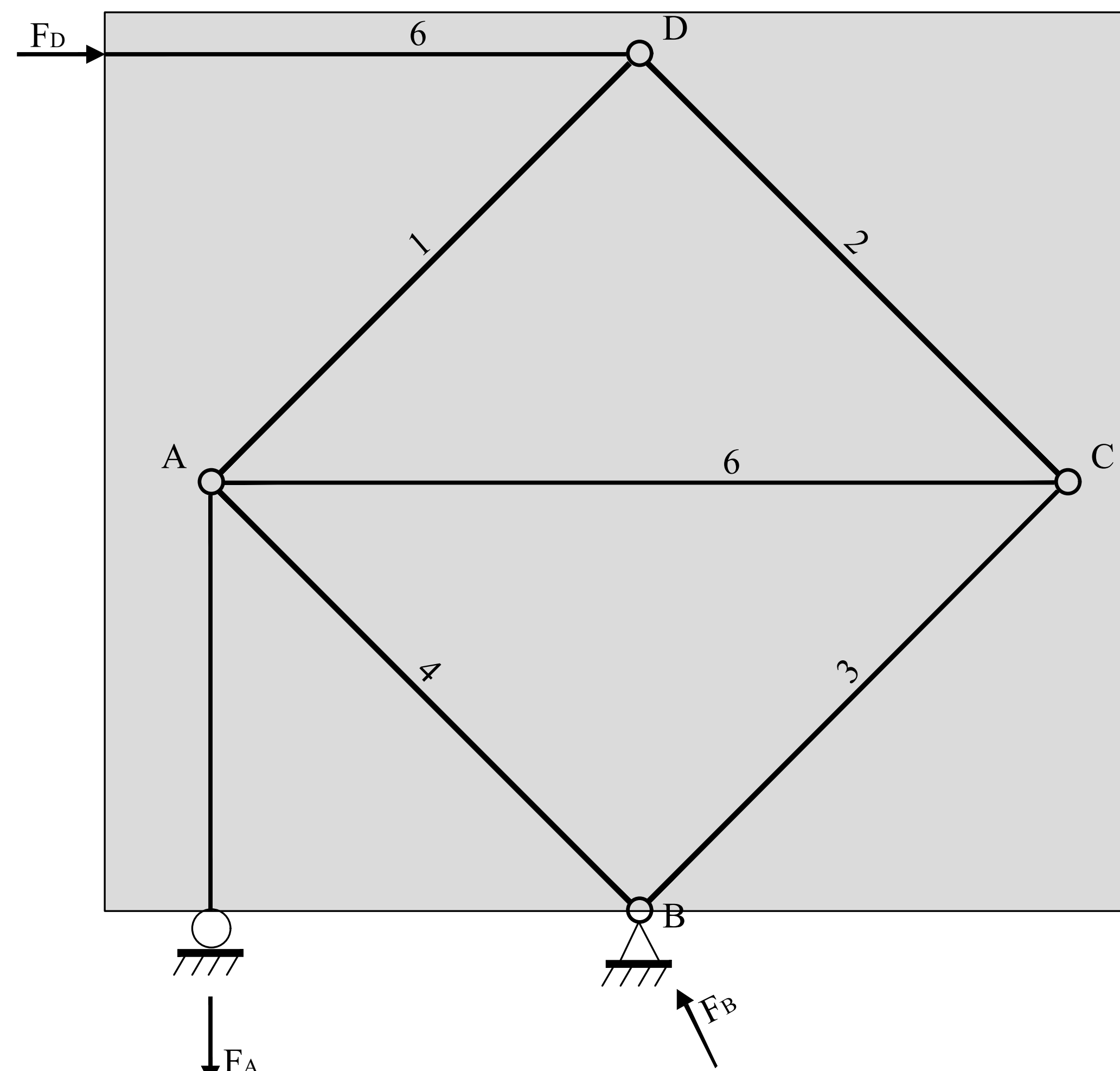
DIAGRAMME DES SITUATIONS
