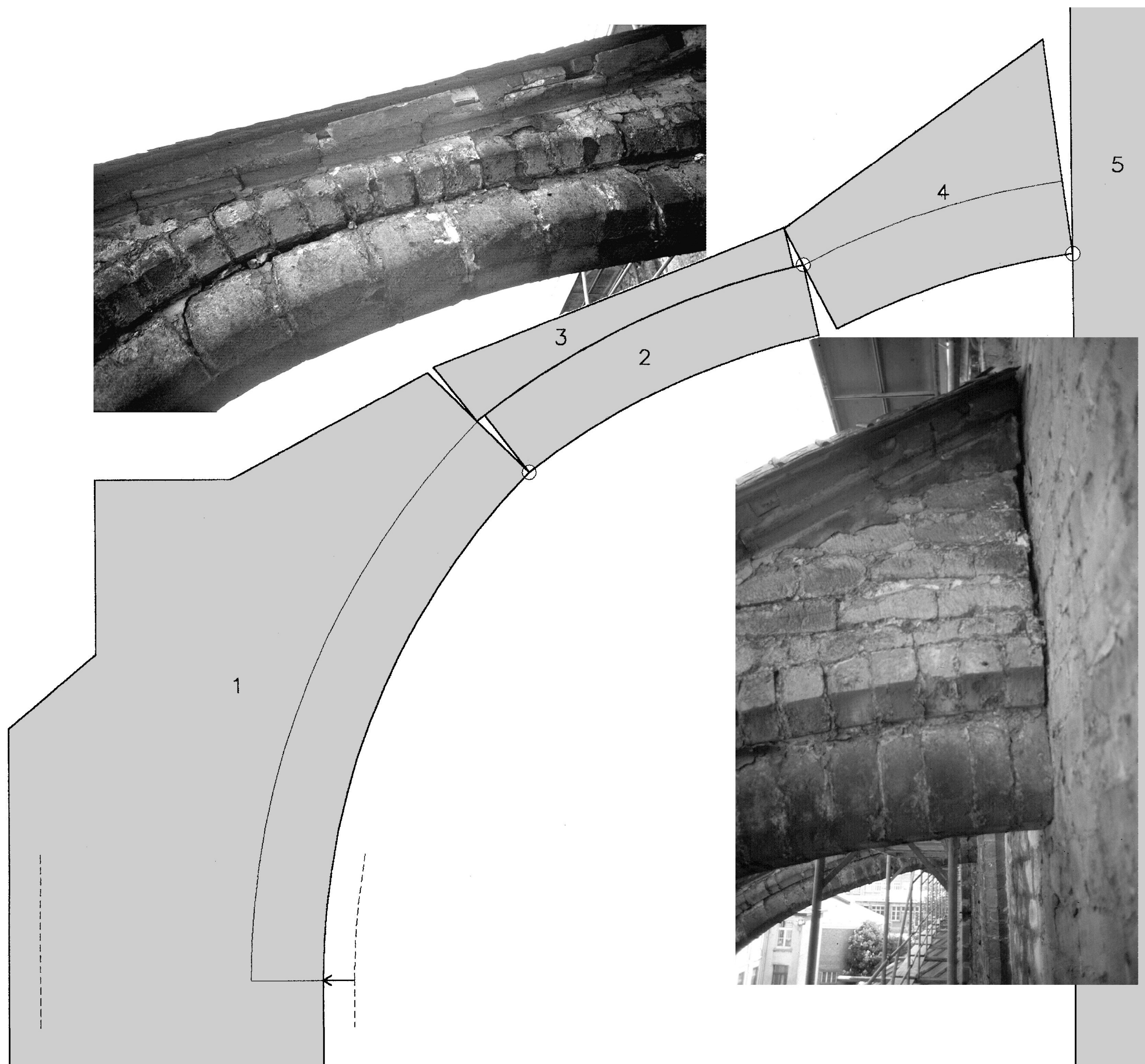
Fig. 50 : Arc-boutant de l'église ND aux Dominicains à Leuven (schéma)
