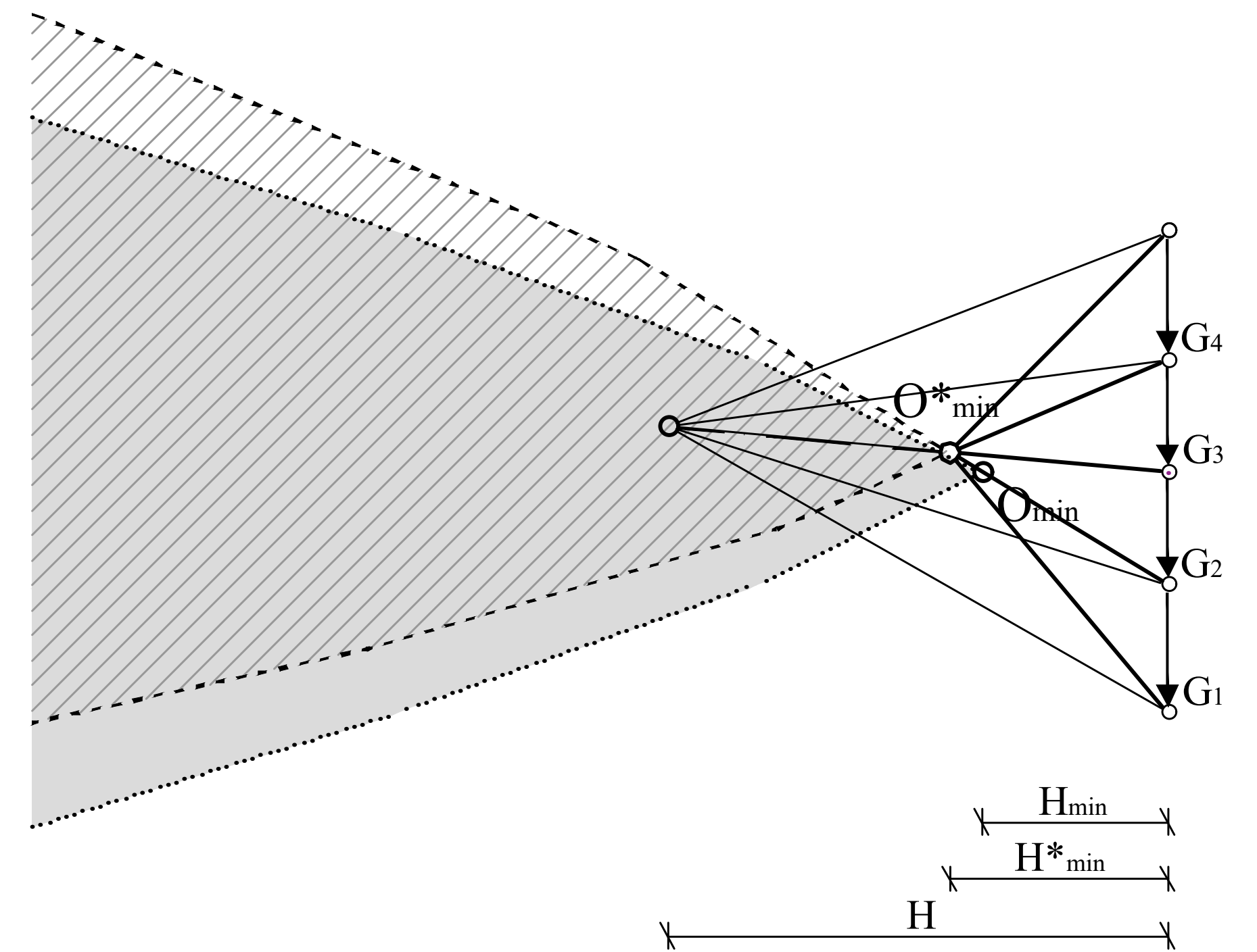
Diagramme des forces [k]
