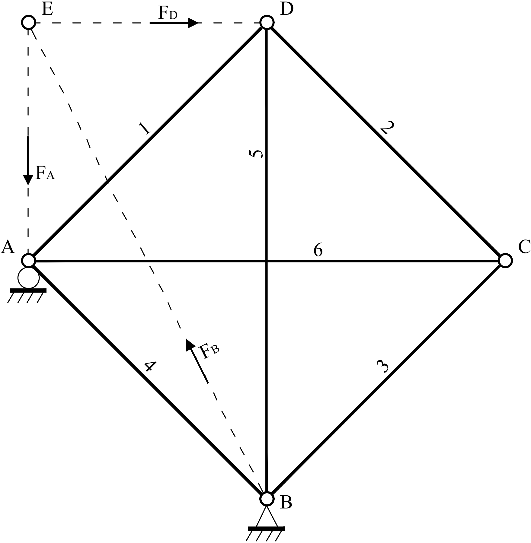
DIAGRAMME DES SITUATIONS
