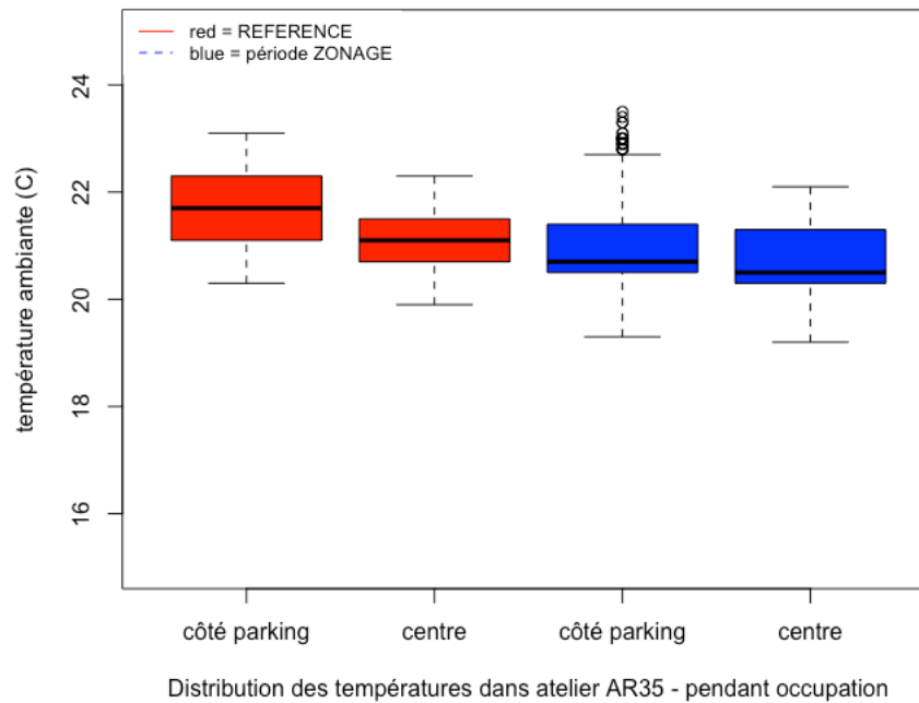
Figure 32 Distribution des températures dans l'atelier Master 2 AR35, selon les périodes d'expérience, en période d'occupation. Les périodes VOLONTAIRE et STOP n'ont pas pu être mesurées (mauvaise manipulation des sondes)
