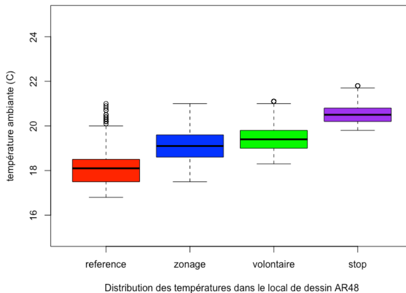
Figure 43 Distribution des températures dans la salle de dessin AR48, selon les périodes d'expérience
