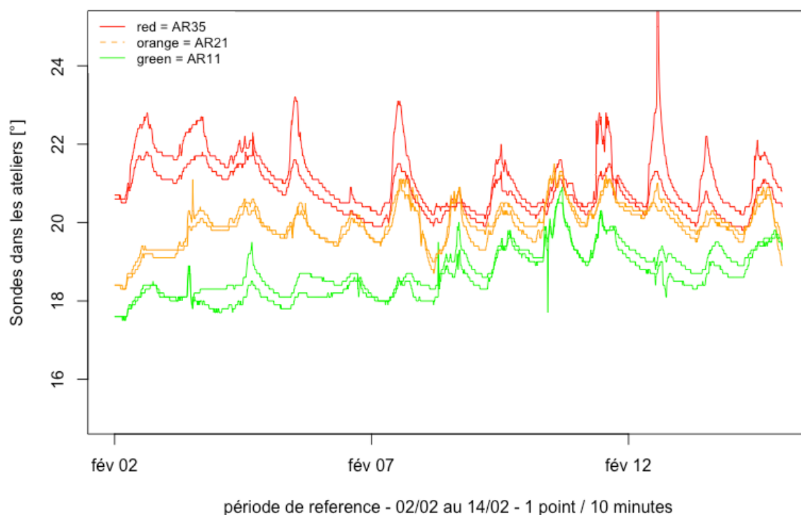
Figure 17 Évolution des températures dans les ateliers pendant la période de référence.
