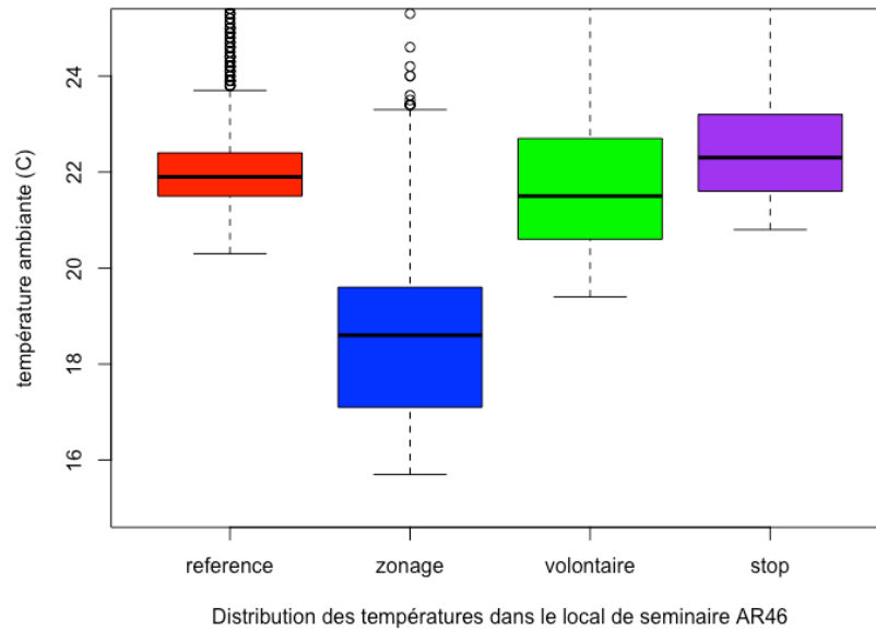
Figure 42 Distribution des températures dans la salle de séminaire AR46, selon les périodes d'expérience
