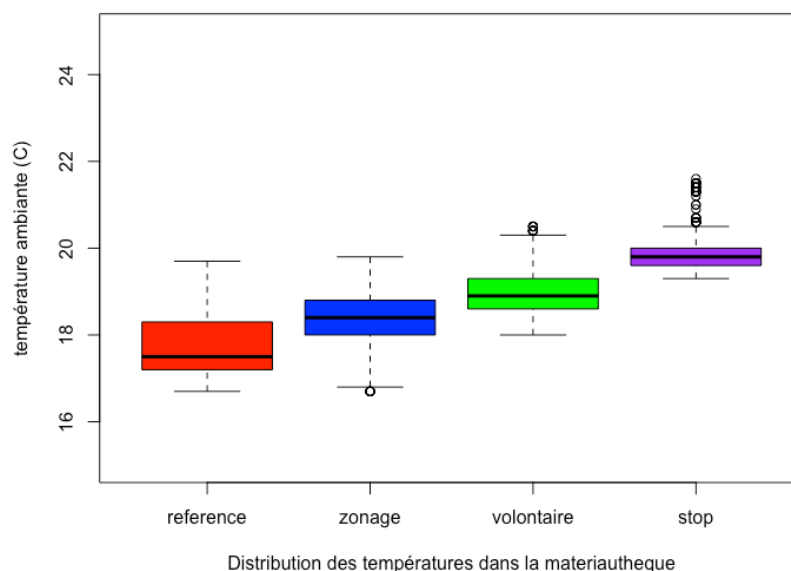
Figure 48 Distribution des températures dans la matériauthèque AR23, selon les périodes d'expérience
