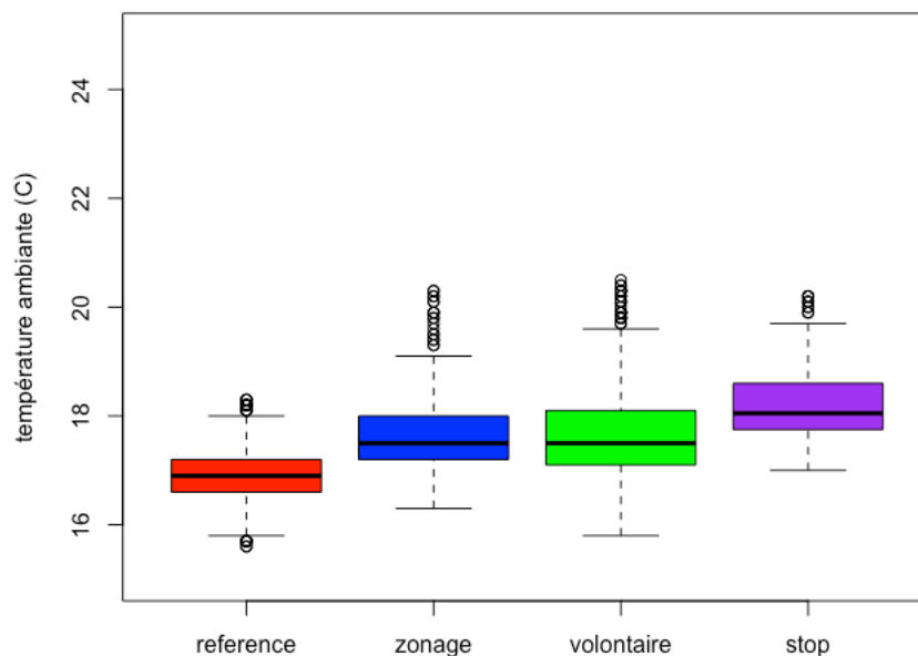
Distribution des températures dans le local enseignants BAC AR12 - pendant occupation
