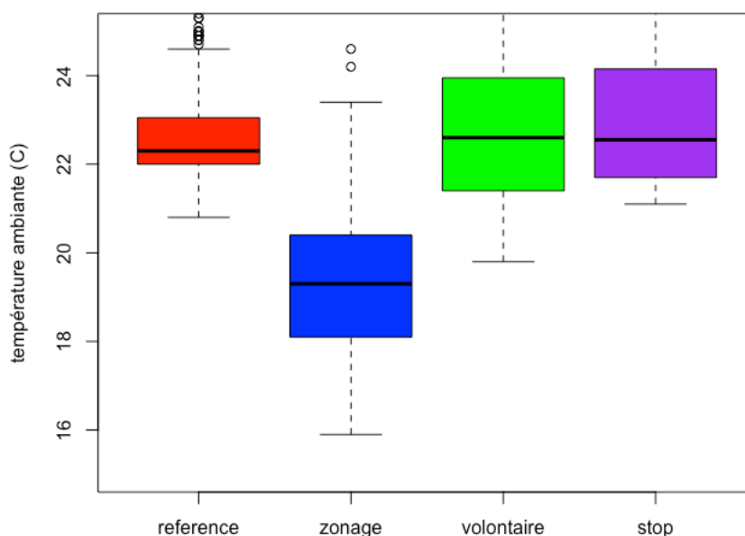
Distribution des températures dans le local de séminaire AR46 - pendant occupation
