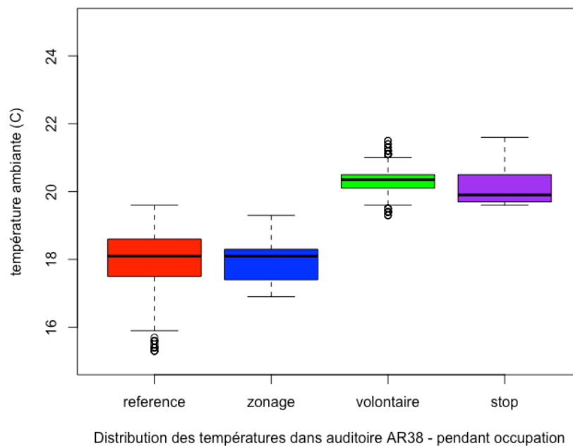
Figure 39 Distribution des températures dans l'auditoire AR38, selon les périodes d'expérience, pendant l'occupation
