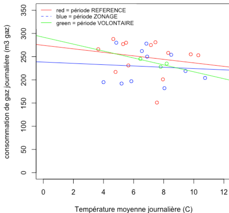
Figure 12 Consommation quotidienne de gaz comparée à la température moyenne journalière, par période
