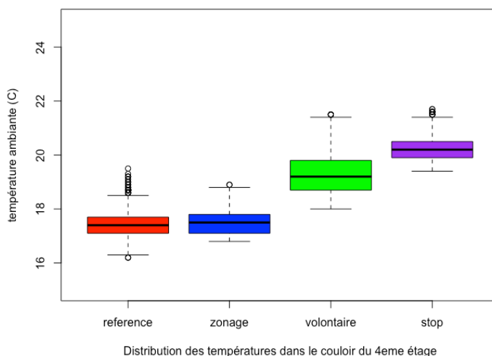
Figure 20 Distribution des températures dans le couloir du 4 ème étage, par période d'expérience.
