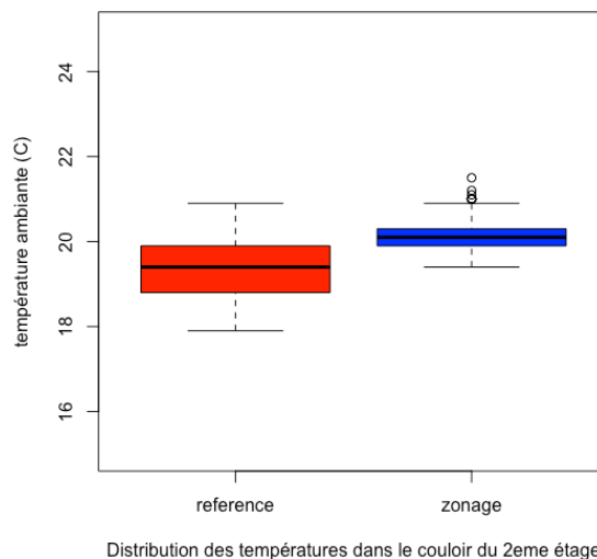
Figure 19 Distribution des températures dans le couloir du 2 ème étage, par période d'expérience. Les périodes VOLONTAIRE et STOP n'ont pas pu être mesurée (vol de sonde)
