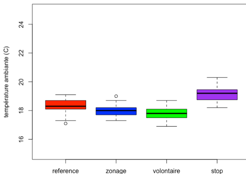
Distribution des températures dans escalier principal - pendant occupation
