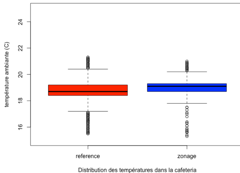
Figure 51 Distribution des températures dans la cafeteria, selon les périodes d'expérience. Les périodes VOLONTAIRE et STOP n'ont pas pu être mesurée (vol de sonde).
