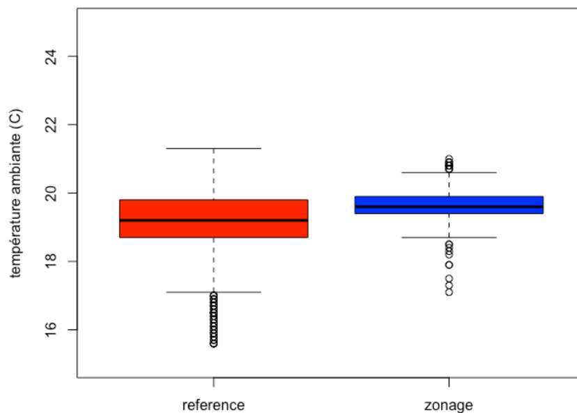
Distribution des températures dans la cafeteria - pendant occupation
