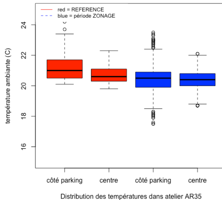
Figure 29 Distribution des températures dans l'atelier Master 2 AR35, selon les périodes d'expérience. Les périodes VOLONTAIRE et STOP n'ont pas pu être mesurées (mauvaise manipulation des sondes)
