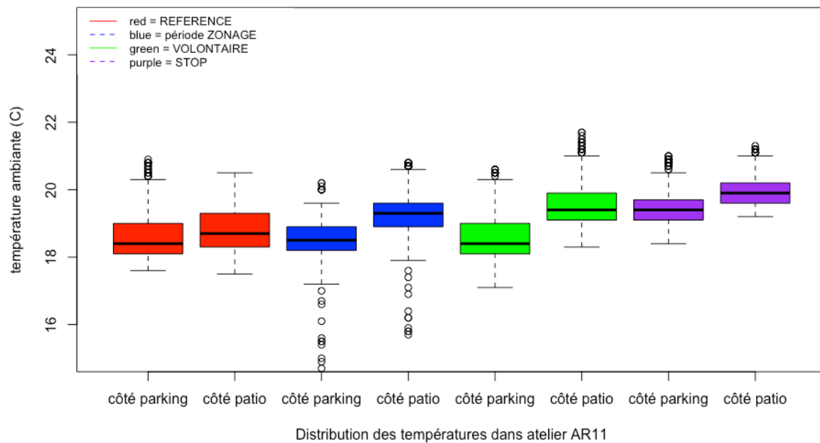
Figure 30 Distribution des températures dans l'atelier BAC AR11, selon les périodes d'expérience.
