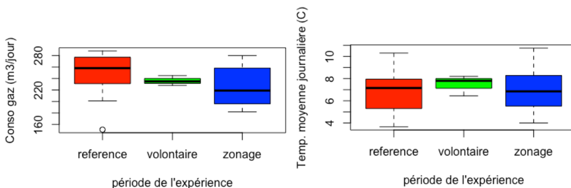
Figure 13 Plages de consommations d'énergie par période d'expérience, en regard des températures extérieures sur la période. Attention, les valeurs pour la période VOLONTAIRE ne portent que sur 3 jours et sont donc peu fiables.
