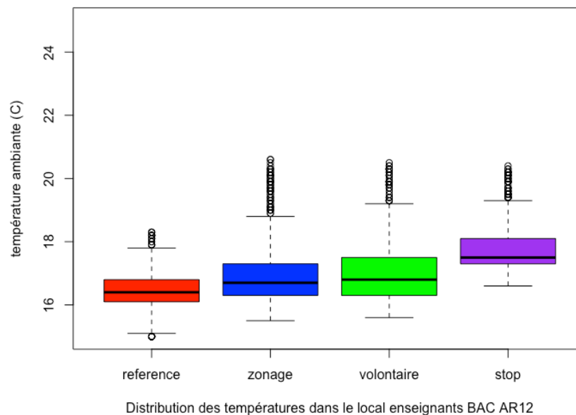
Figure 50 Distribution des températures dans le local d'enseignants master AR12, selon les périodes d'expérience.
