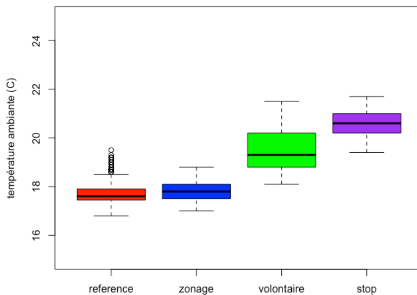
Distribution des températures dans le couloir du 4eme étage - pendant occupation
