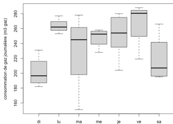
Figure 10 Distribution des consommations par jour de la semaine, pour toute la période relevée
