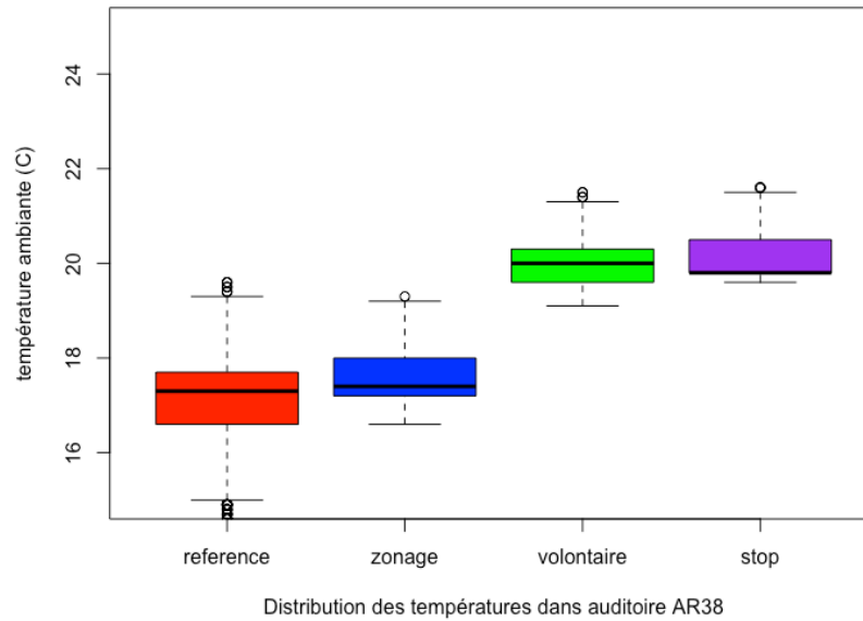
Figure 38 Distribution des températures dans l'auditoire AR38, selon les périodes d'expérience
