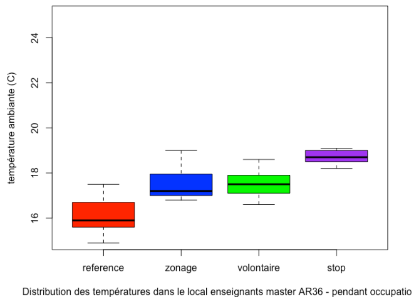
Figure 53 Distribution des températures dans le local d'enseignants master AR36, selon les périodes d'expérience, pendant l'occupation.
