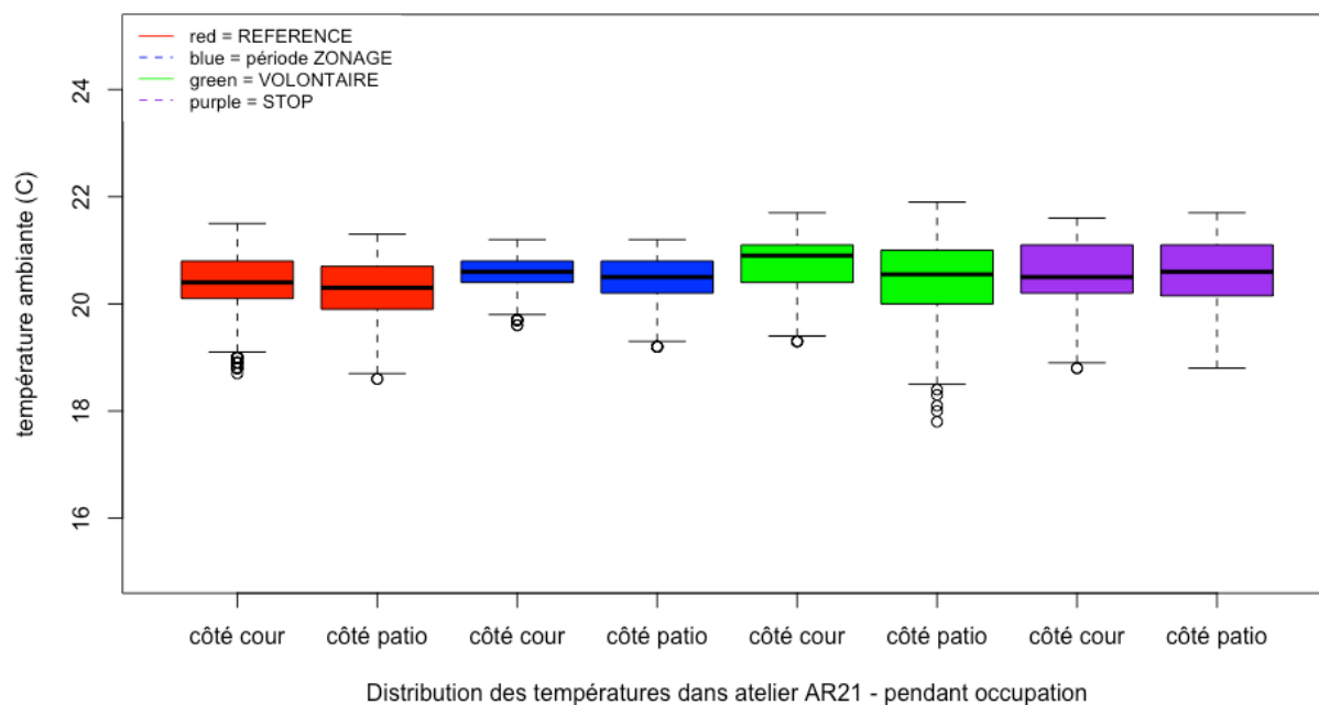
Figure 34 Distribution des températures dans l'atelier MASTER AR21, selon les périodes d'expérience, en période d'occupation
