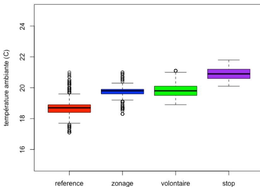
Figure 44 Distribution des températures dans la salle de séminaire AR46, selon les périodes d'expérience, pendant l'occupation
