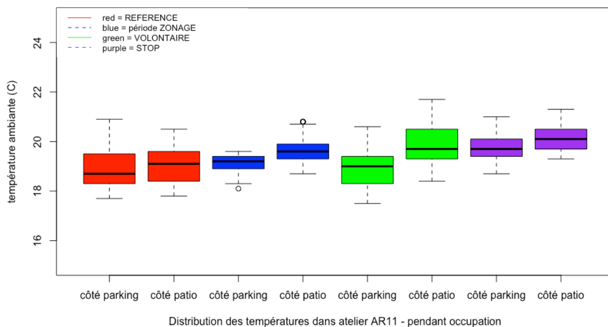
Figure 33 Distribution des températures dans l'atelier BAC AR11, selon les périodes d'expérience, en période d'occupation.
