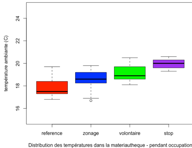
Figure 52 Distribution des températures dans la matériauthèque AR23, selon les périodes d'expérience, pendant l'occupation
