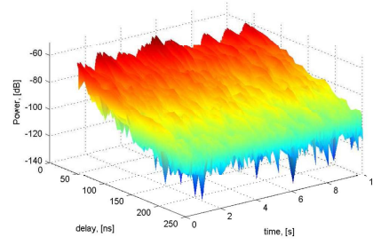
(d) Measured time-variant PDP, node Rx7
