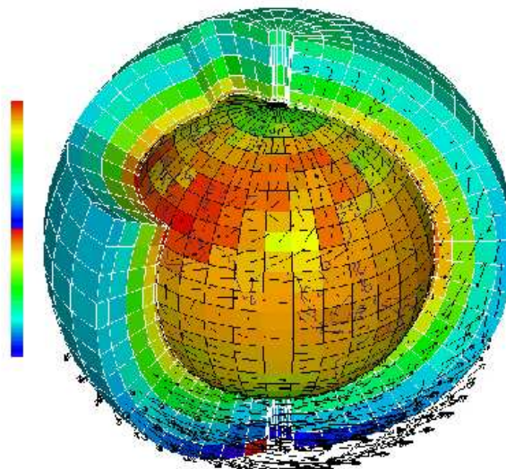
Figure 11 : Maillage tri-dimensionnel d'un modèle de simulation du climat
