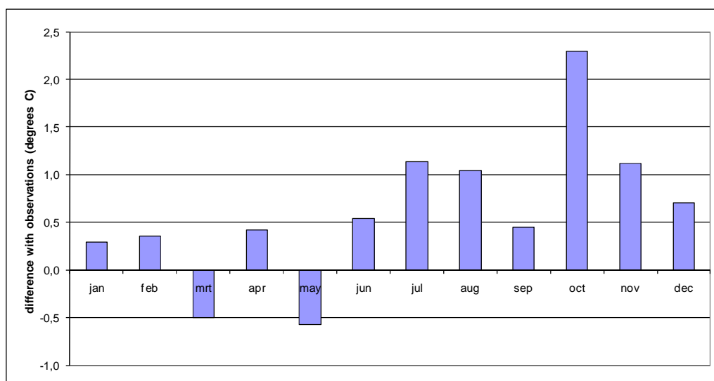
Figure 19 : Différence mensuelle entre les températures observées et simulées, moyenne sur cinq stations météorologiques, moyenne des modèles
