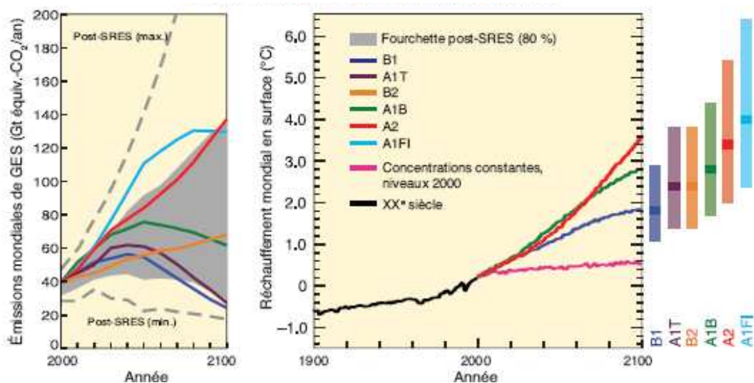
Figure 9 : Scénarios d'émissions de GES pour la période 2000-2100 (en l'absence de politiques climatiques additionnelles) et projections relatives aux températures en surface
