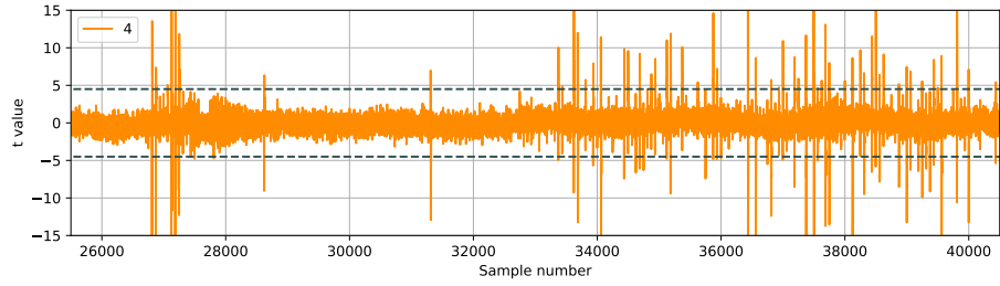
(b) Exemplary t -test on EM traces for byte 4.
