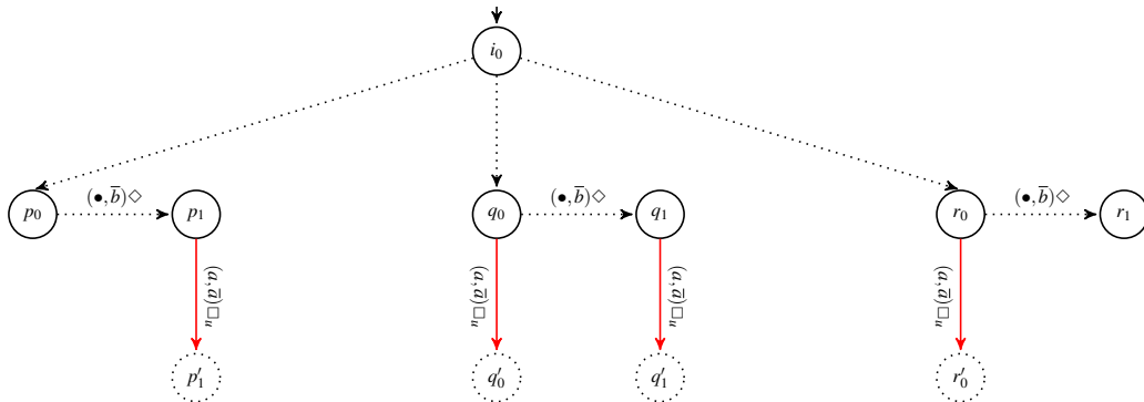
Fig. 10: Automaton \mathcal{A}'
