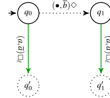
Fig. 9: Automaton \mathcal{A}
