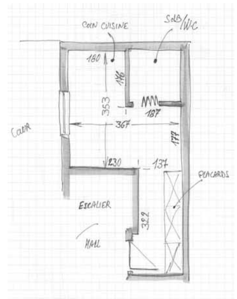
Plan d'un petit logement à Mons — P. Roucou SPW DG04
