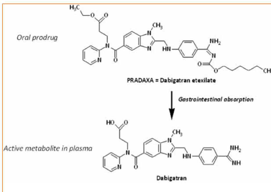
Figure 1 : Structure moléculaire du dabigatran éxétilate (Pradaxa®) et conversion en son métabolite actif, le dabigatran.
