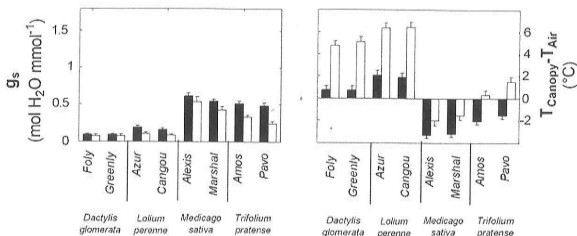
FIGURE 4 : Conductance stomatique ( g_s ) en fonction des différentes espèces et différence entre la température foliaire ( T_{\text{canopy}} ) et la température de l'air ( T_{\text{air}} ) pour ces mêmes espèces. Une valeur négative indique une température foliaire inférieure à la température de l'air. Une valeur positive indique une température foliaire supérieure à celle de l'air, et donc un échauffement de la surface foliaire.
