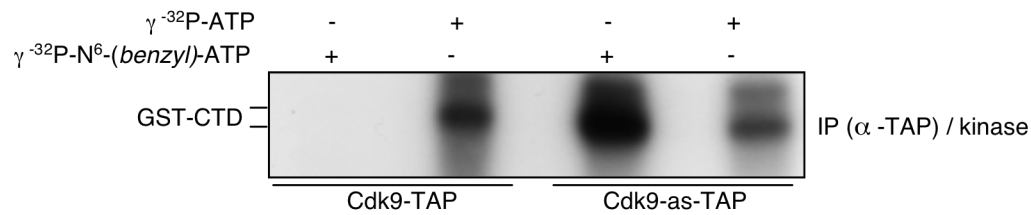
Figure 14. Utilisation spécifique du ^{32}\text{P} -N 6 -(benzyl)-ATP par la protéine « analogue sensible » Cdk9-as. Des cellules de S. pombe exprimant l'allèle intégratif cdk9-TAP ou cdk9-as-TAP ont été lysées pour immunoprécipiter les protéines Cdk9-TAP et Cdk9-as-TAP en utilisant des billes magnétiques coatées d'anticorps dirigés contre le tag TAP. L'activité kinase sur le substrat GST-CTD a été testée lors d'une réaction kinase in vitro utilisant soit le \gamma - ^{32}\text{P} -ATP ou le \gamma - ^{32}\text{P} -N 6 -(benzyl)-ATP, suivie d'un gel SDS-PAGE et d'une autoradiographie.
