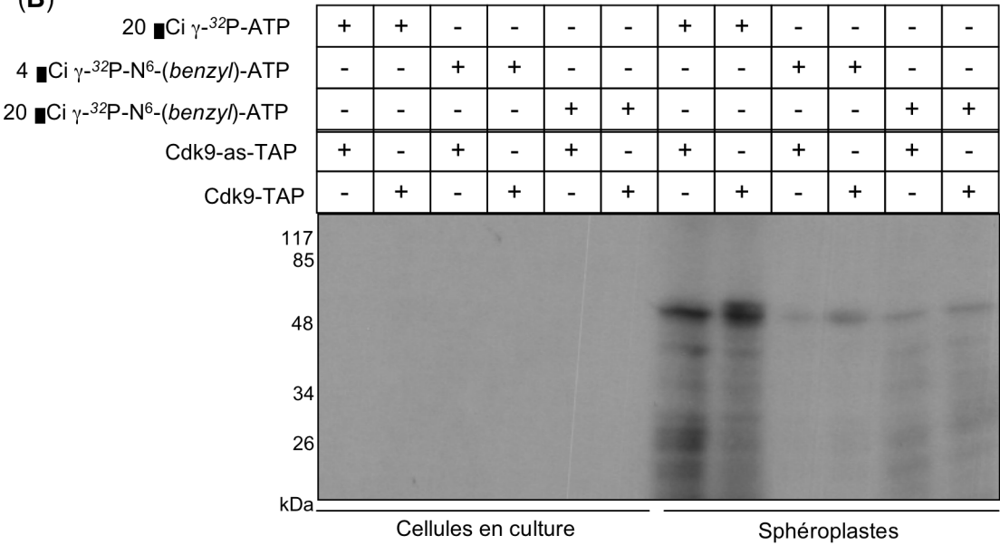
Figure 10. Phosphorylation inexistante ou aspécifique des substrats des kinases -as dans un extrait cellulaire. (A) Test kinase in vivo réalisé avec 10 µCi de \gamma - 32 P-ATP sur 100 µg d'extrait protéique obtenu à partir d'une souche S. pombe sauvage. Variation de la composition du tampon de réaction kinase : présence ou absence d'1 mM d'ATP froid, 1 mM de DTT ou d'inhibiteurs de protéases. L'histone H1 devant a priori être phosphorylée par la kinase Cdc2 de l'extrait protéique nous sert de contrôle. La phosphorylation d'une bande aux environs de 50 kDa est détectée dans la majorité de nos tests in vivo peu importe les conditions ou les souches utilisées. Elle est considérée comme aspécifique. (B) Test kinase in vivo réalisé avec les quantités en \gamma - 32 P-ATP et \gamma - 32 P-N 6 -(benzyl)-ATP mentionnées dans la figure sur les souches cdk9-TAP et cdk9-as-TAP . Les cellules ont été cultivées en milieu progressivement appauvri en phosphate (6 h en EMM 1 mM NaH 2 PO 4 puis de 20 h en EMM 50 µM NaH 2 PO 4 ) et le test kinase a été effectué sur des cellules en culture (ajout des sources d'ATP radioactif dans le milieu de culture) ou sur des sphéroplast (ajout des sources d'ATP radioactif après digestion de la paroi des cellules à la zymolyase). Pour ces deux figures, le poids moléculaire des protéines de l'étalon est affiché à gauche.
