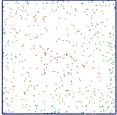
(d) Re_\tau = 300 , \rho_p/\rho = 1000 , F_{el}/F_g = 0.026
