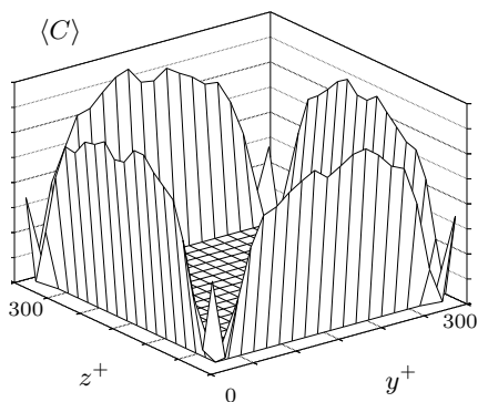
(d) Re_\tau = 300 , \rho_p/\rho = 1000 , F_{el}/F_g = 0.026
