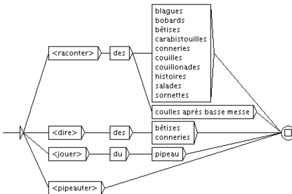
Figure 1 : exemple de graphe complexe UNITEX
