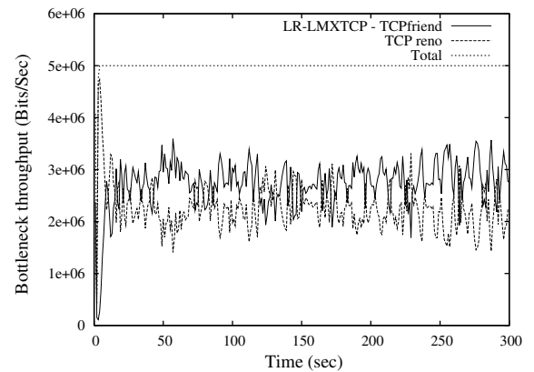
(b) LR-LMXTCP-TCPfriend
