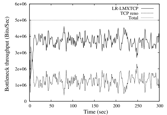
(a) LR-LMXTCP
