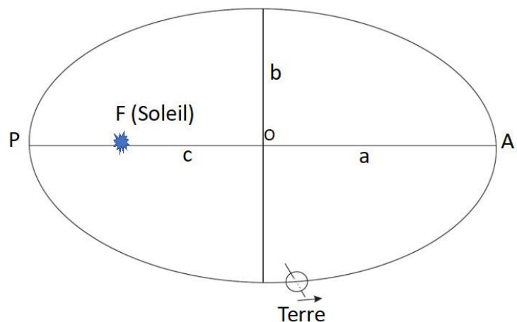
Figure 2. Orbite elliptique de la Terre autour du Soleil. O est ...
