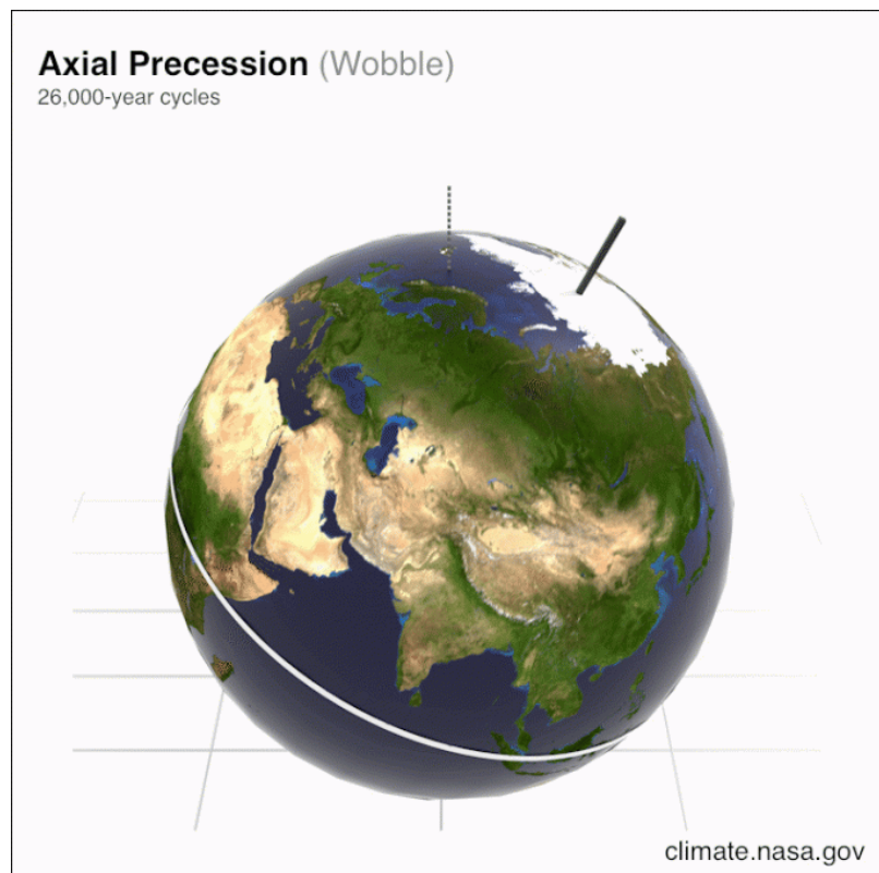
Figure 5. Animation représentant la précession astronomiq...
