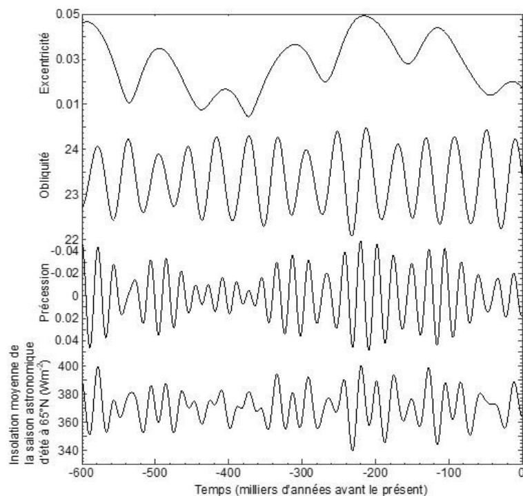
Figure 11. Variations à long terme sur les derniers 600 000 a...
