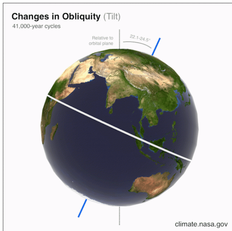
Figure 3. Animation représentant les modifications de l'obli...
