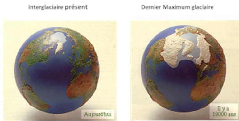
Figure 1. L'extension des glaces de l'hémisphère nord aujourd'hui...
