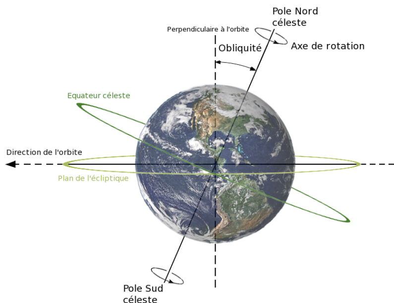
Figure 4. L'écliptique et sa relation avec l'équateur céleste et...
