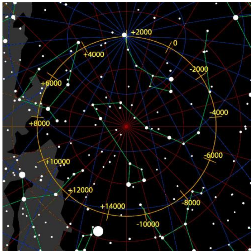
Figure 6. Précession astronomique. Parcours du Pôle Nord ...
