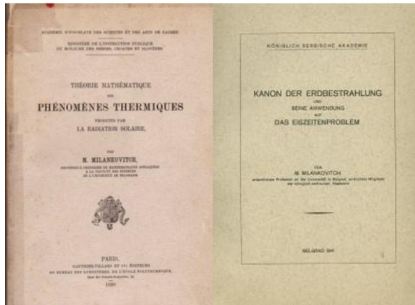
Figure 8. Couvertures des deux livres de Milankovitch. [Sour...
