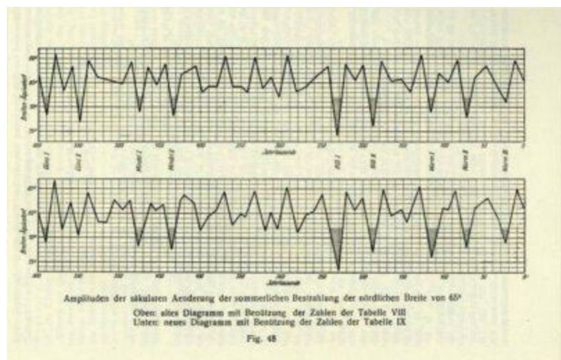
Figure 10. Variations à long terme de la latitude équivalente...
