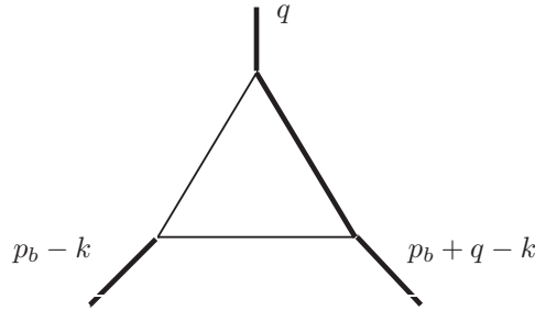
Figure 5.16: Triangle n.1: t_1
