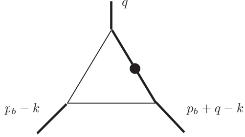
(a) Triangle n.2: t_2
