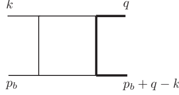
Figure 5.21: Box n.1: box_1
