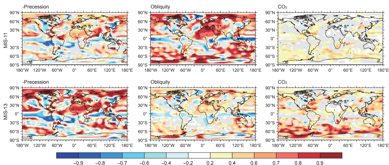
图 2 LOVECLIM模拟的MIS-11和MIS-13时期全球年降水与负岁差、斜率和CO 2 的多元线性回归图 [73] 。灰色阴影区域代表相关系数在统计意义上不显著( P>0.05 )。当岁差越小时,北半球夏季太阳辐射越高;而岁差越大时,北半球夏季太阳辐射越低。为了从太阳辐射的角度来探讨降水和岁差的关系,本文用负岁差来进行多远线性回归分析
