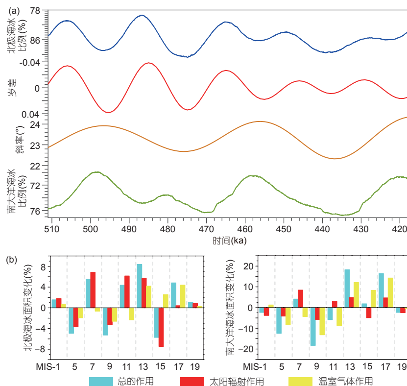
图 1 北极和南大洋海冰变化 [19,20] . (a) 轨道驱动下LOVECLIM模拟的北极和南大洋年均海冰变化 [19] 及其与岁差和斜率 [59] 的对比. 从上到下依次为: 北极海冰比例、岁差、斜率、南大洋海冰比例. (b) 太阳辐射和温室气体对过去80万年每个间冰期北极和南大洋年均海冰变化单独和总的作用. 海冰面积变化(%)是与参考实验相比较 [20]
