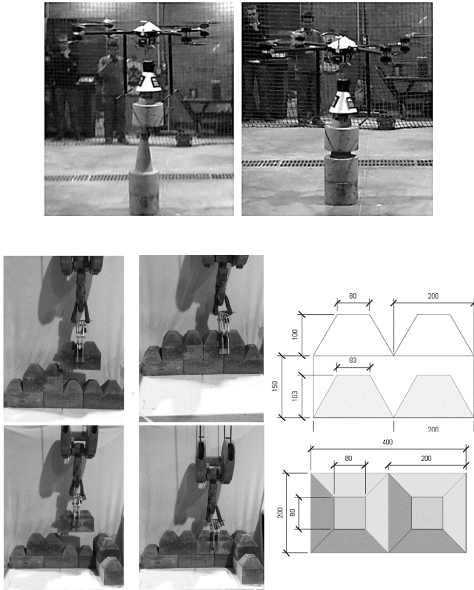
Figure 2 : quelques exemples des blocs de maçonnerie « drone compatible » développés à l'UCL dans le cadre du projet de recherche.
