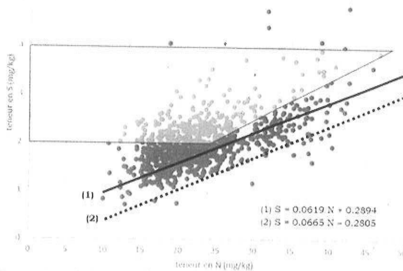
FIGURE 3 : Teneurs en azote et soufre des fourrages wallons et seuils de carence phytotechnique (lignes continues et pointillées) et zootechnique (surface grisée) Figure 3 : Nitrogen and sulfur content of Walloon forages and phytotechnical (solid and dotted lines) and zootechnical (shaded area) deficiency thresholds.
