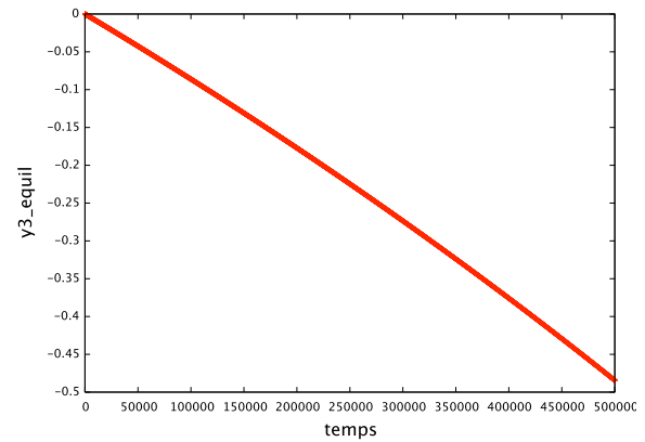
FIG. 10.18 – Evolution de la valeur d'équilibre de y_3 en fonction du temps exprimé en années.
