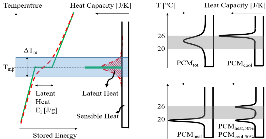
Figure 2. (a) Propriétés des PCM dans la courbe Enthalpie/Température et la capacité calorifique associée. Comportement idéal (vert) et quasi-idéal (ligne rouge discontinue). (b) Comparaison conceptuelle de la solution à deux PCM et à un PCM.
